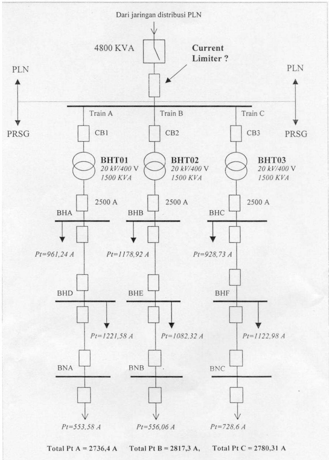
Gambar 1. Diagram satu garis sistem kelistrikan RSG-GAS yang disederhanakan.
