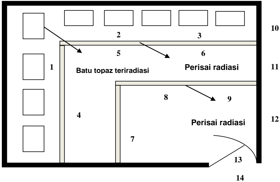
Gambar 2. Denah bagian dalam ruang penyimpanan batu topaz sementara dan titik pengukuran
