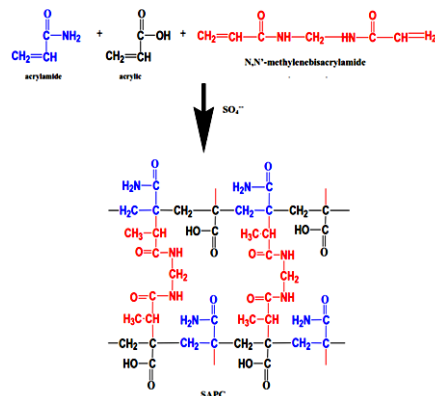
Gambar 2. Reaksi kimia pembuatan Polimer Super Absorbent [8]
