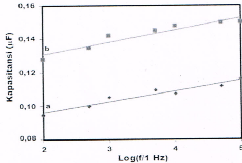
Gambar 5. Nilai kapasitansi (a) mikro komposit dan (b) nano-komposit Fe_{0,5}-C_{0,5}
