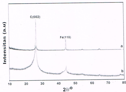
Gambar 1. Pola XRD serbuk komposit Fe_{0,5}-C_{0,5} (a) sebelum dan (b) sesudah proses milling selama 50 jam
