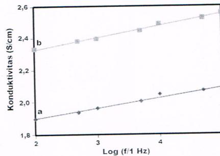
Gambar 4. Nilai konduktivitas (a) mikrokomposit dan (b) nano-kompisit Fe_{0,5}-C_{0,5}
