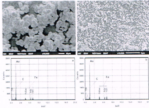
Gambar 2. Morfologi permukaan serbuk komposit Fe-C (a) sebelum dan (b) sesudah milling selama 50 jam
