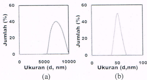
Gambar 3. Distribusi ukuran partikel serbuk komposit Fe_{0,5}-C_{0,5} (a) sebelum dan (b) sesudah proses milling selama 50 jam.
