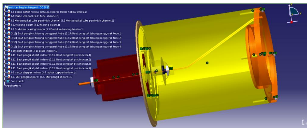
Gambar 3. Gambar hasil perakitan bagian bergerak modul distributor channel
