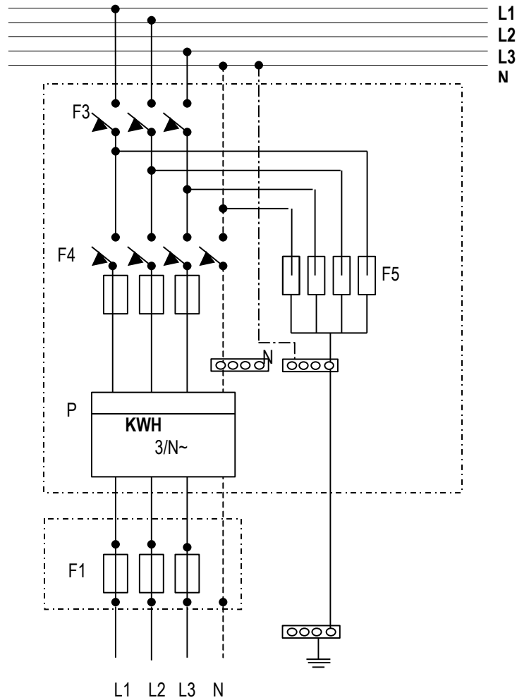
Gambar 7. Diagram rangkain pemasangan instalasi overvoltage arrester
