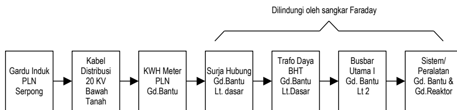
II. METODOLOGI Gambar 5. Diagram balok urutan aliran listrik ke RSG-GAS
