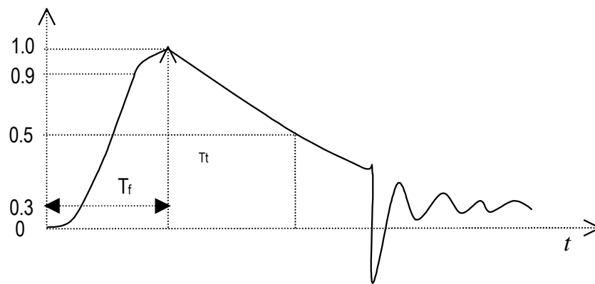
Gambar 1. Bentuk umum gelombang impuls petir
