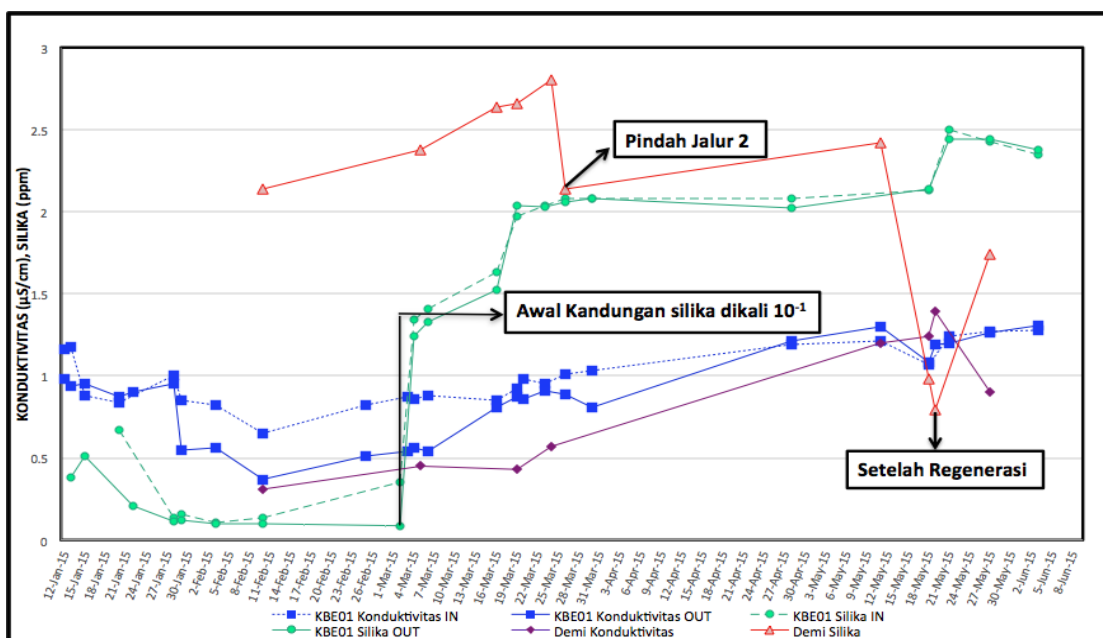
Gambar 4.1 :Grafik hasil pengukuran konduktivitas air dan kandungan silika dalam air pendingin primer sebelum dan sesudah melewati sistem pemurnian air kolam reaktor(KBE01)serta dalam air bebas mineral
