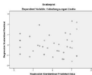
Gambar 3. Uji Heteroskedastisitas
