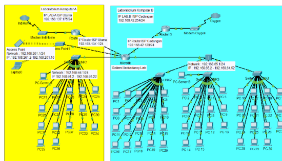
Gambar 3. Topologi Jaringan Usulan
