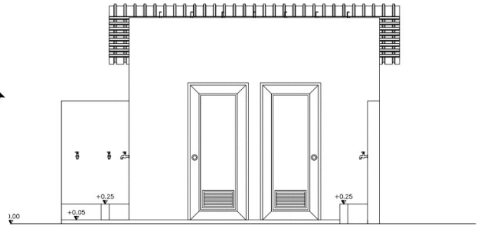
Gambar 15. Gambar tampak depan kamar mandi baru
