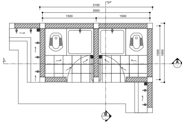
Gambar 14. Gambar denah kamar mandi baru
