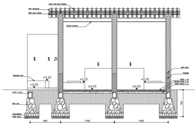
Gambar 16. Gambar potongan memanjang kamar mandi baru
