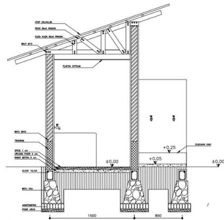
Gambar 17. Gambar potongan melintang kamar mandi baru
