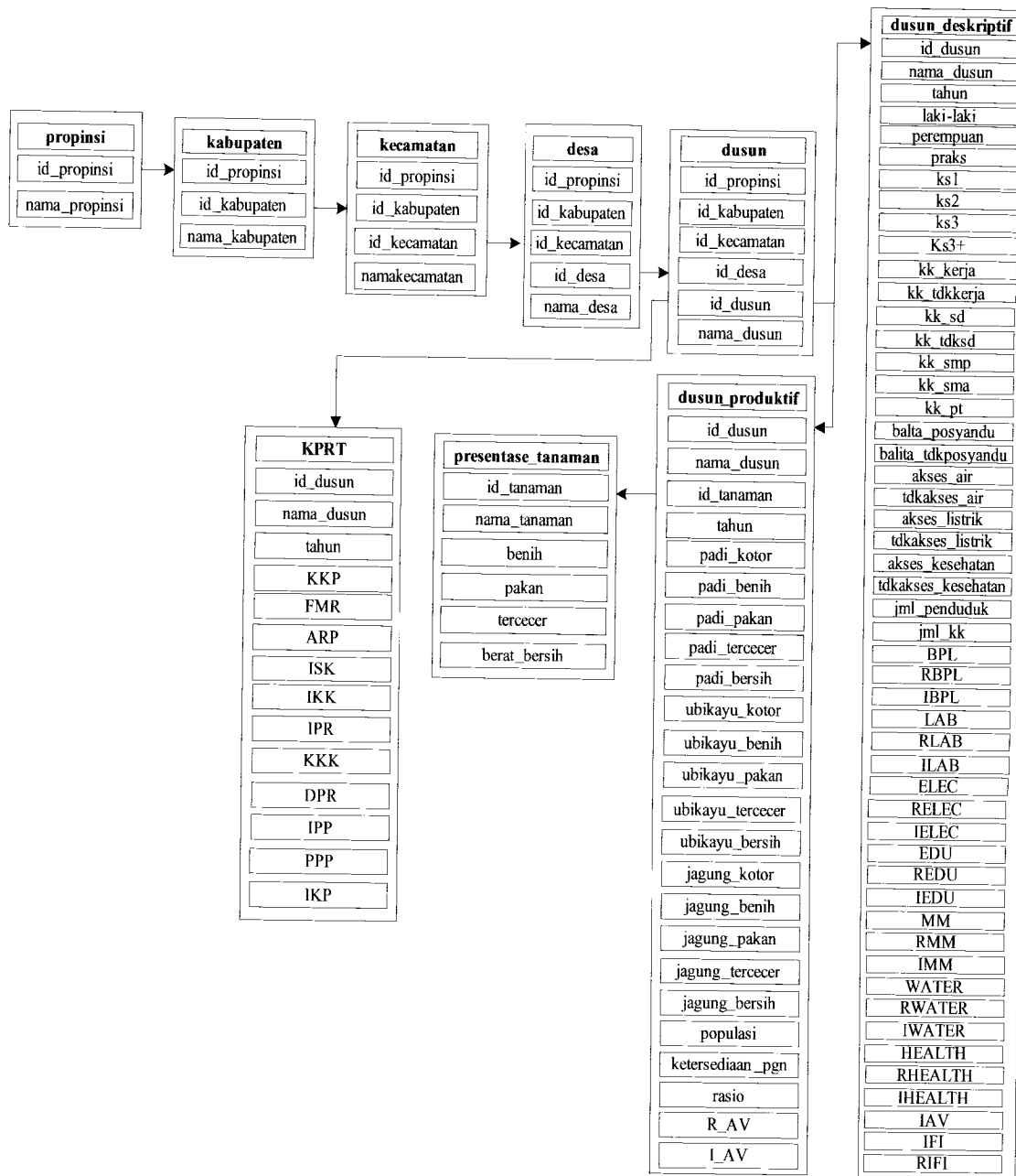
Gambar 7. Manajemen subsistem basis data SPK untuk penetapan indeks ketahanan pangan
