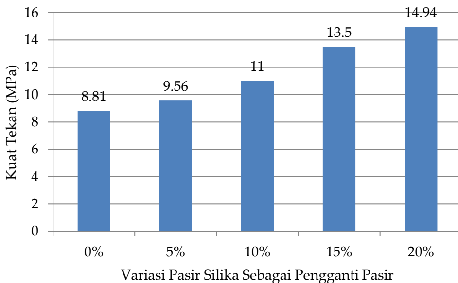
Gambar 4. Hubungan Variasi Pasir Silika dan Kuat Tekan Rata-Rata Paving Block
