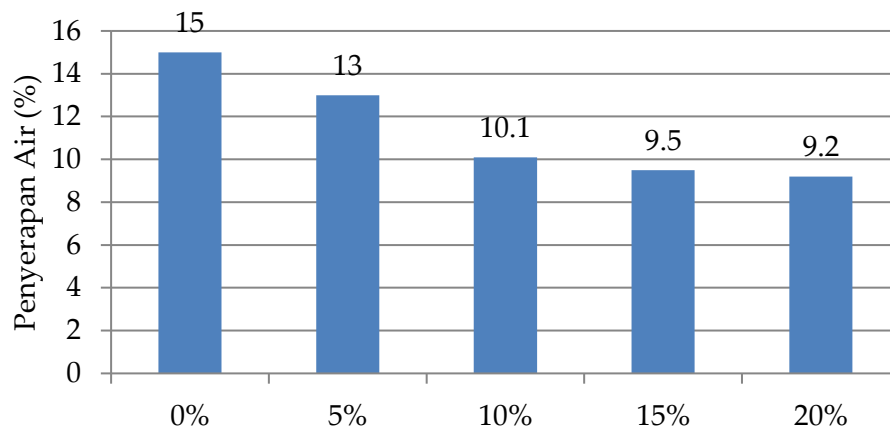
Gambar 5. Hubungan Variasi Pasir Silika dan Penyerapan Air Rata-Rata Paving Block
