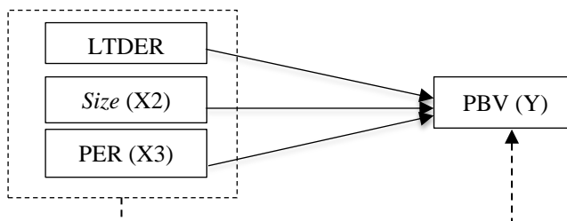
Gambar 1. Kerangka Teoritik
