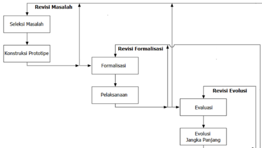
Gambar 4. Model siklus hidup sistem pakar oleh Rolston [79]
