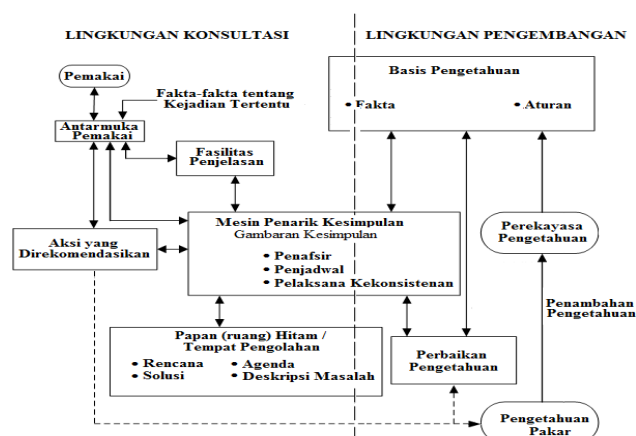
Gambar 1. Struktur lengkap sebuah sistem pakar
