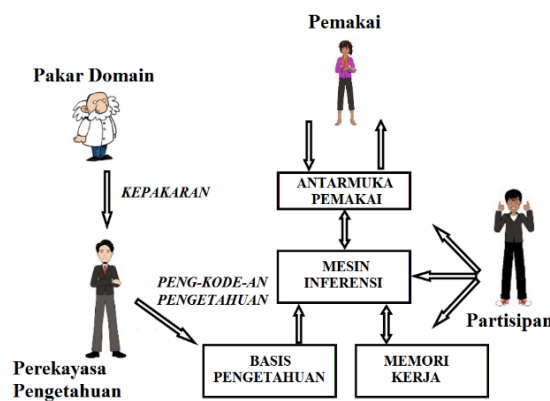
Gambar 2. Komponen sistem pakar
