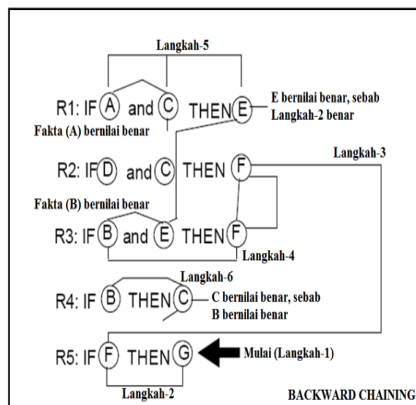
Gambar 3. Runut mundur: Pencocokan fakta atau pernyataan dimulai dari bagian sebelah kanan (THEN)
