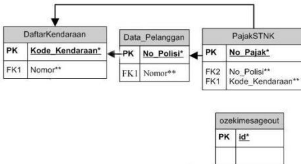
Gambar 6. Rancangan Database
