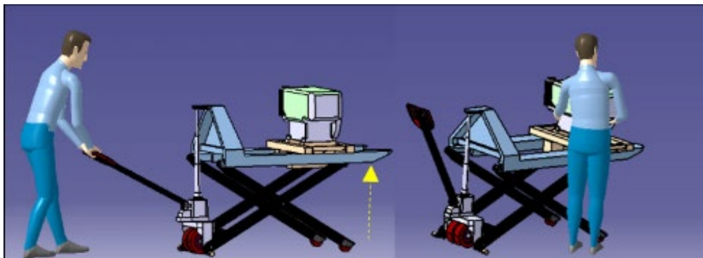
Gambar 8. Simulasi pada kegiatan peletakan mesin diesel (Sumber: CATIA V5)
