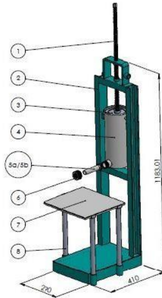
Gambar 1. Mesin pengolah sosis kapasitas 50 kg/jam
