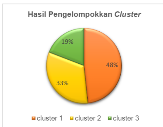
Gambar 8. Diagram Lingkaran
