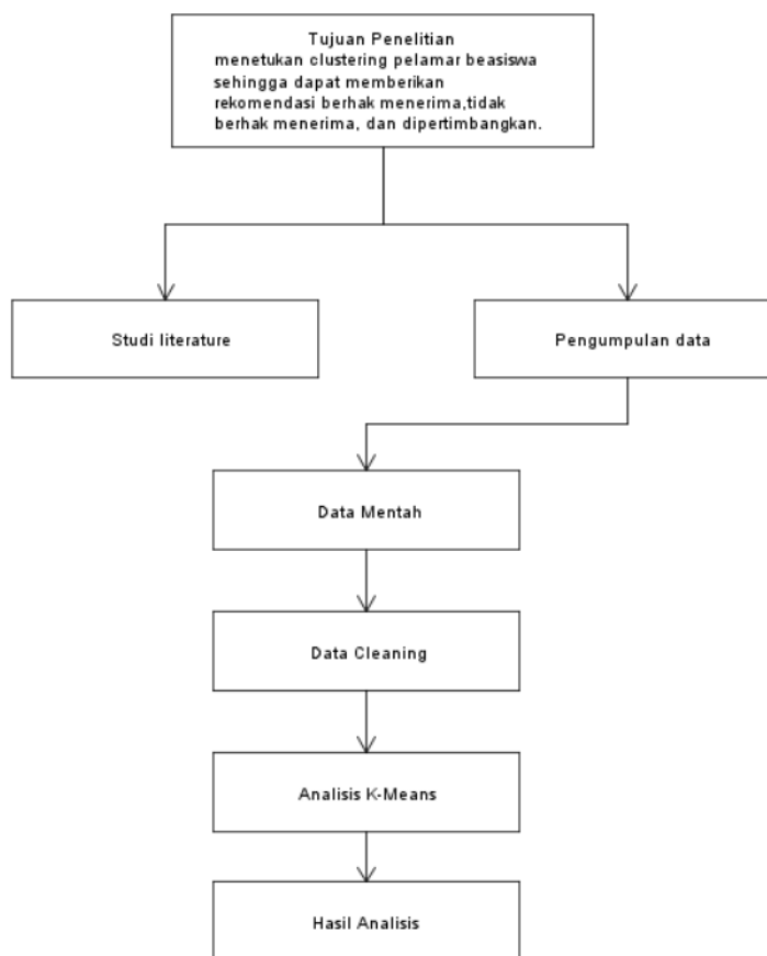
Gambar 1. Tahapan Penelitian
