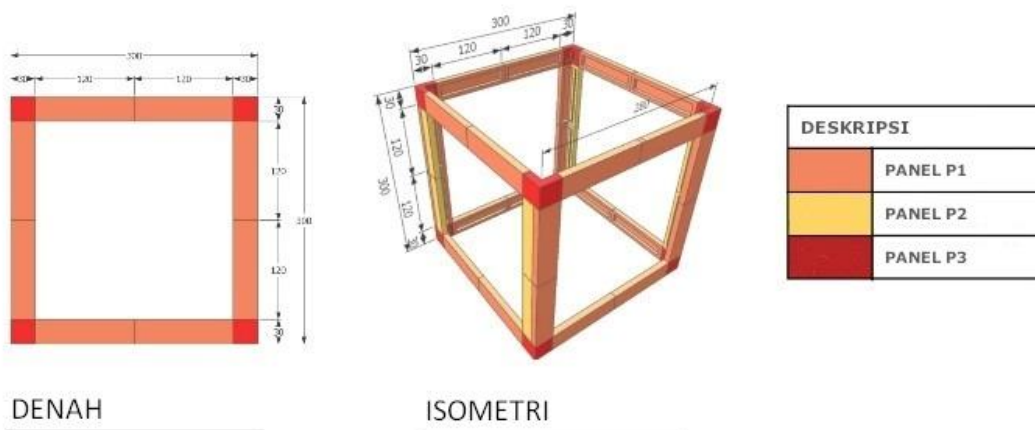
Gambar 1. Modul RISHA [5]
