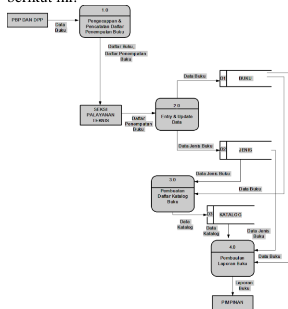
Gambar 4. Data Flow Diagram (DFD) Level 0 Sistem Pengolahan Data Katalog pada Perpustakaan Umum Muhammad Hatta
