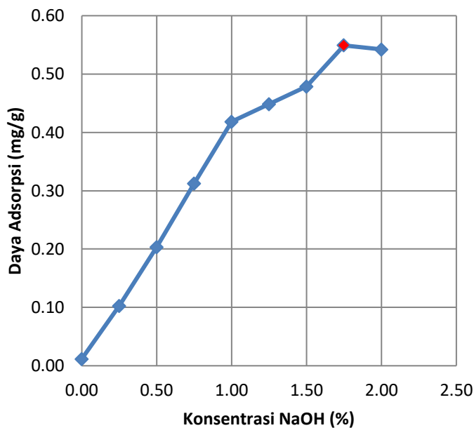
Gambar 1. Grafik Hubungan Antara Daya Serap (mg/g) Arang Aktif Tongkol Jagung terhadap Ion Pb^{2+} pada berbagai Variasi Konsentrasi.
