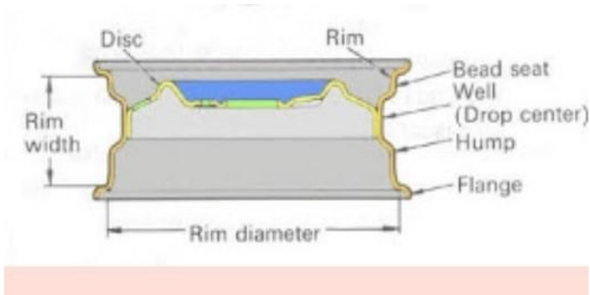
Gambar 3. Konstruksi velg.
