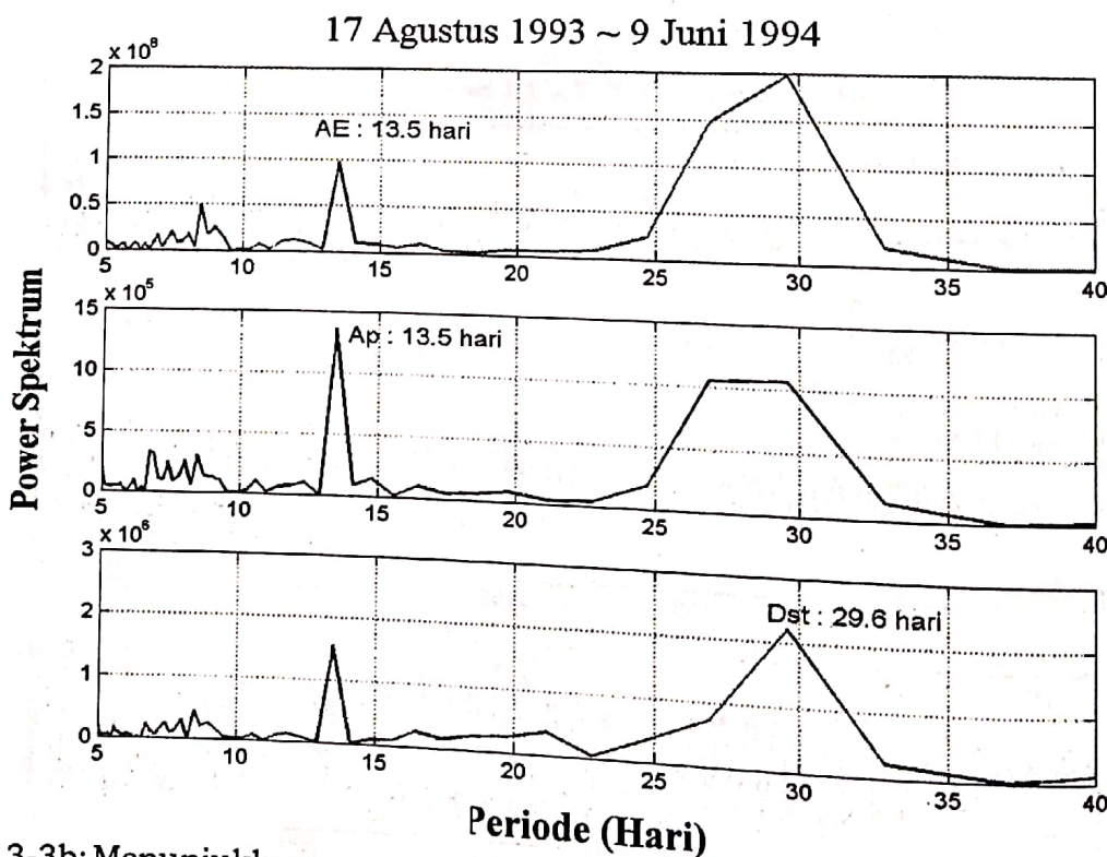
Gambar 3-3b: Menunjukkan power spectrum indeks magnet global Dst, AE, Ap pada tanggal 17 Agustus 1993 sampai dengan tanggal 9 Juni 1994
