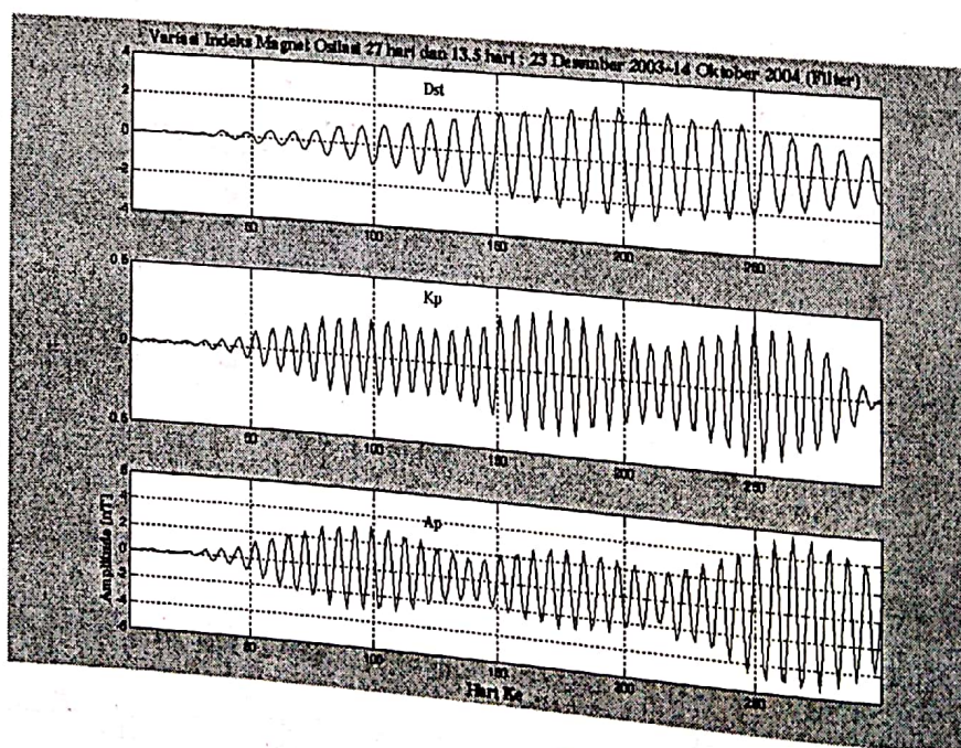
Gambar 3-4c: Menunjukkan variasi osilasi indeks magnet pada tanggal 23 Desember 2003 sampai dengan tanggal 14 Oktober 2004
