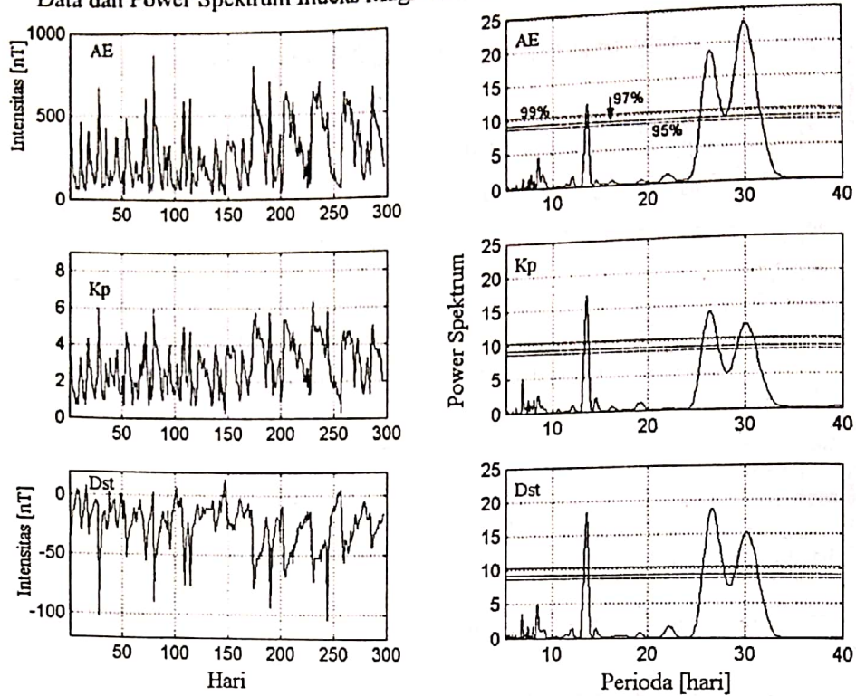
Gambar 3-7: Variasi indeks geomagnet global : AE (lintang tinggi), Kp (lintang tengah) dan Dst (lintang rendah) seperti terlihat pada sebelah kiri, serta fluktuasi power spektrum terhadap periode (kanan) tanggal 17 Agustus 1993 sampai 09 Juni 1994. Garis mendatar menunjukkan tingkat signifikansi puncak spektrum dengan masing-masing peluang adalah 99%, 97% dan 95%
