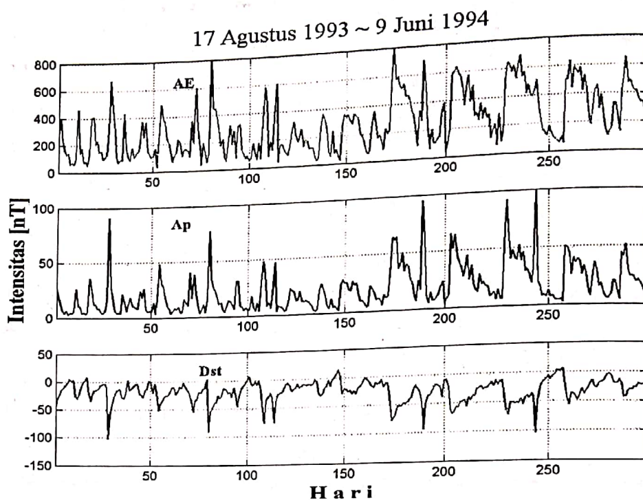
Gambar 3-3a: Variasi indeks magnet global Dst, AE, dan Ap bertepatan dengan aktivitas magnet periodik pada tanggal 17 Agustus 1993 sampai 9 Juni 1994
