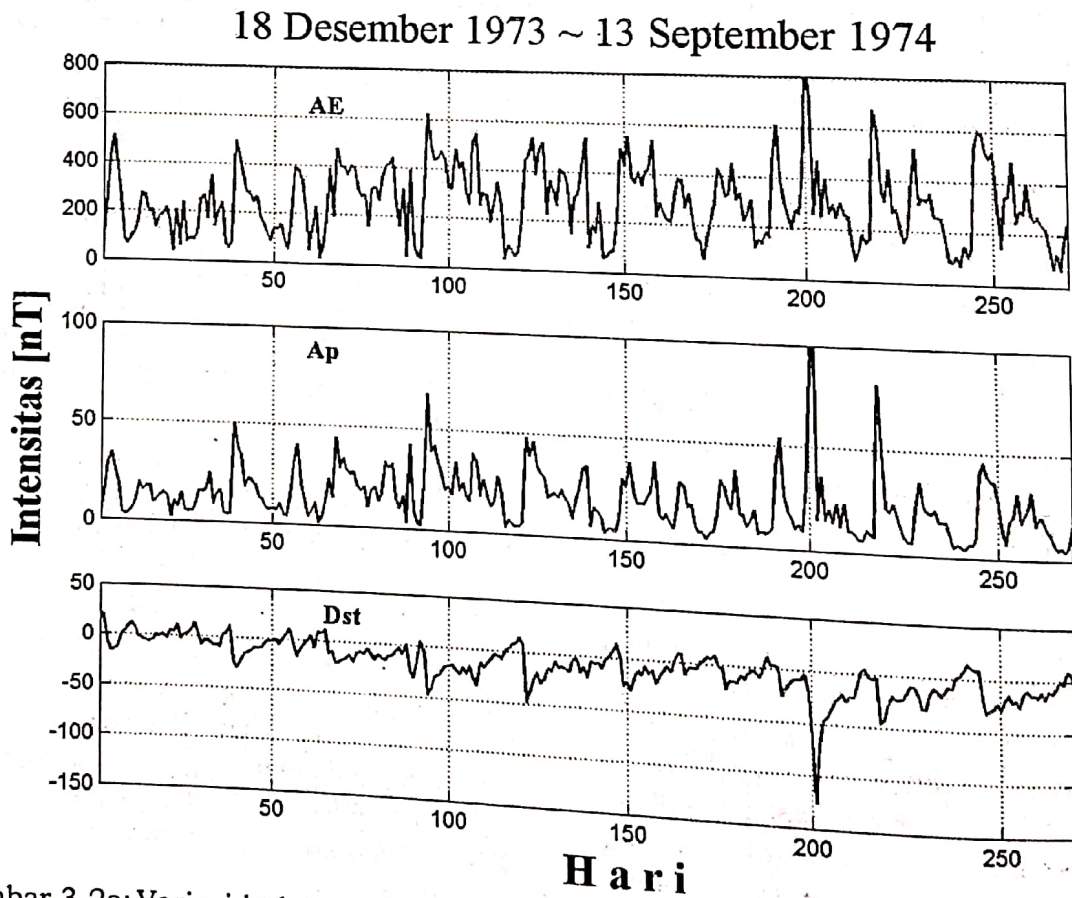
Gambar 3-2a: Variasi indeks magnet global Dst, AE, dan Ap bertepatan dengan aktivitas magnet periodik pada tanggal 18 Desember 1973 sampai 13 September 1974
