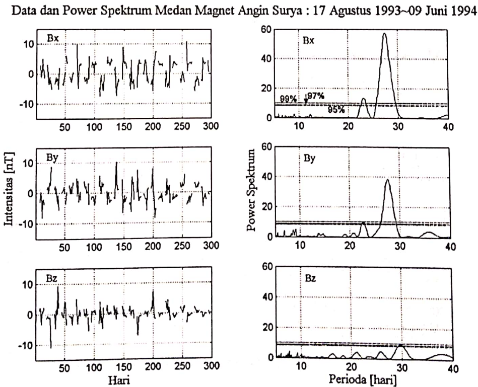
Gambar 3-6: Variasi komponen medan magnet angin surya : B_x , B_y dan B_z (kiri) dan fluktuasi power spektrum terhadap periode (kanan) tanggal 17 Agustus 1993 sampai 09 Juni 1994. Garis mendatar menunjukkan tingkat signifikansi puncak spektrum dengan masing-masing peluang adalah 99%, 97% dan 95%
