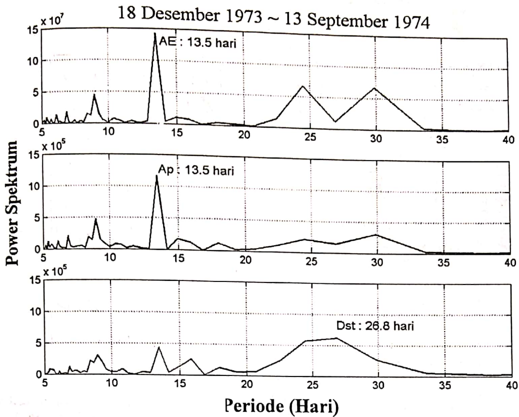
Gambar 3-2b: Menunjukkan power spektrum indeks magnet global Dst, AE, Ap pada tanggal 18 Desember 1973 sampai dengan tanggal 13 September 1974
