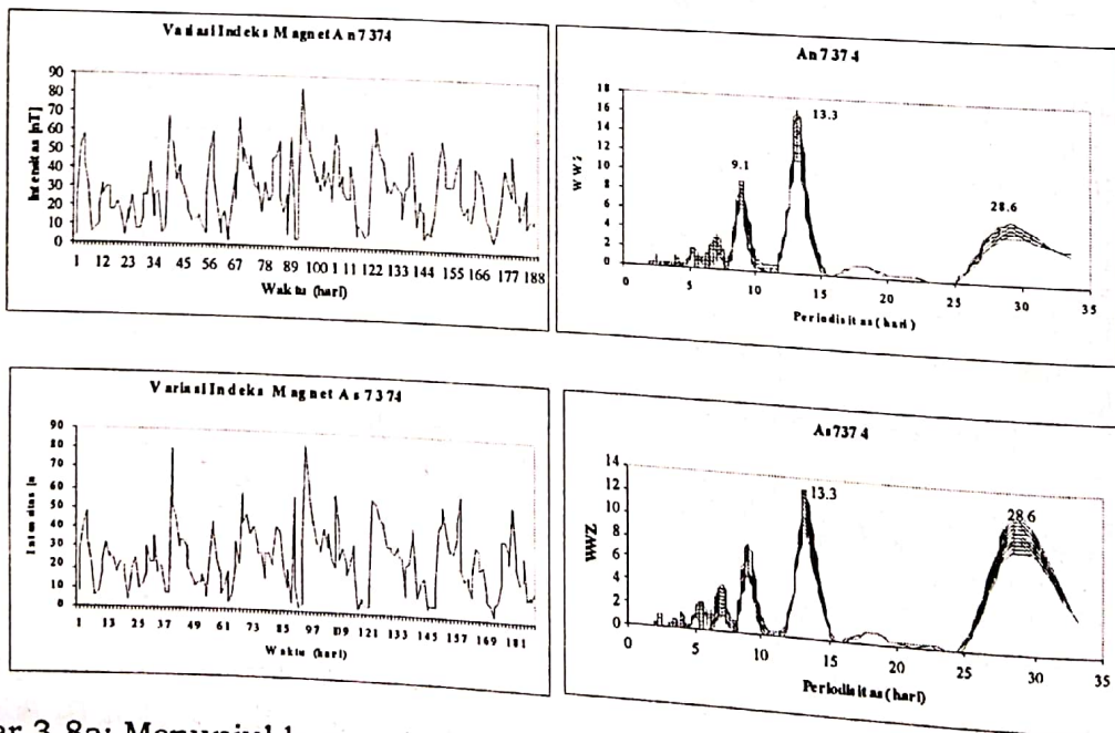
Gambar 3-8a: Menunjukkan variasi dan periodisitas indeks An dan As pada tahun 1973 sampai dengan tahun 1974
