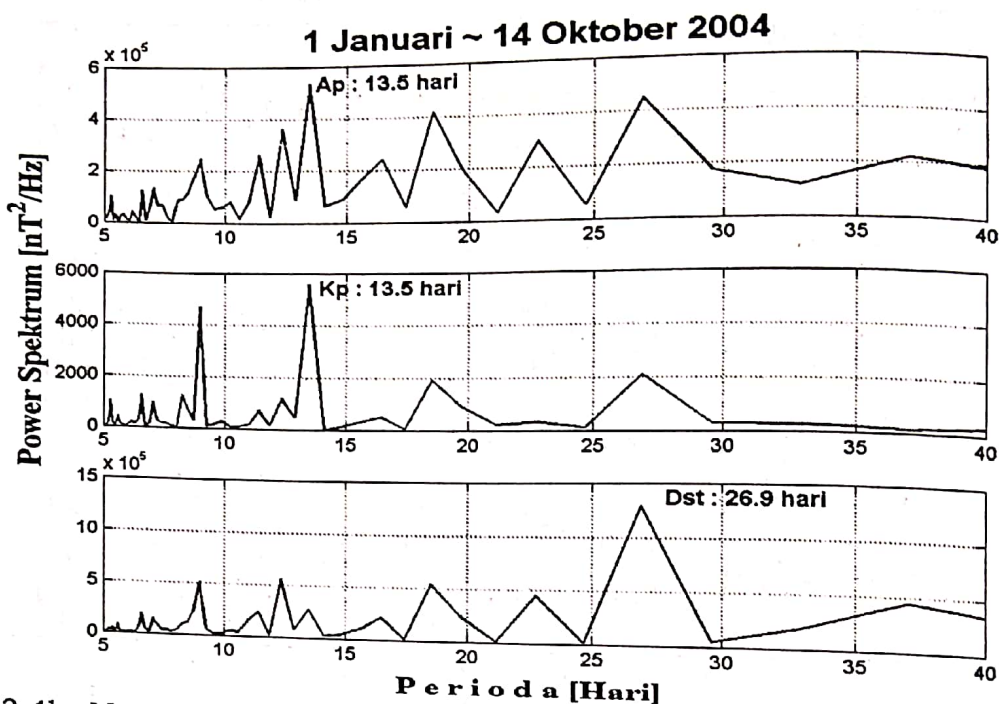
Gambar 3-4b: Menunjukkan power spectrum indeks magnet global Dst, AE, Ap pada tanggal 1 Januari 2004 sampai dengan tanggal 14 Oktober 2004
