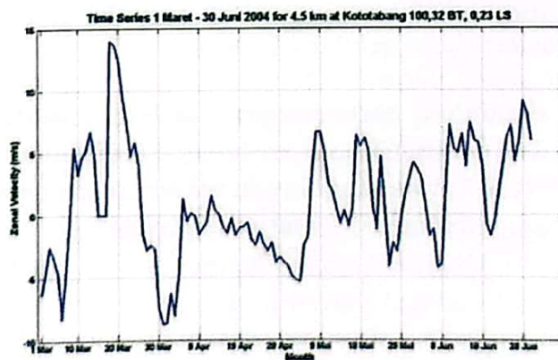
Gambar 4-1d: Time-series angin zonal EAR periode 1 Maret hingga 30 Juni 2004 pada ketinggian 4,5 km
