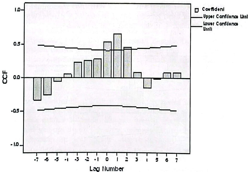
Gambar 4-3a: Grafik korelasi silang OLR-curah hujan (MAWS) Kototabang pada 1 Maret - 30 Juni 2004
