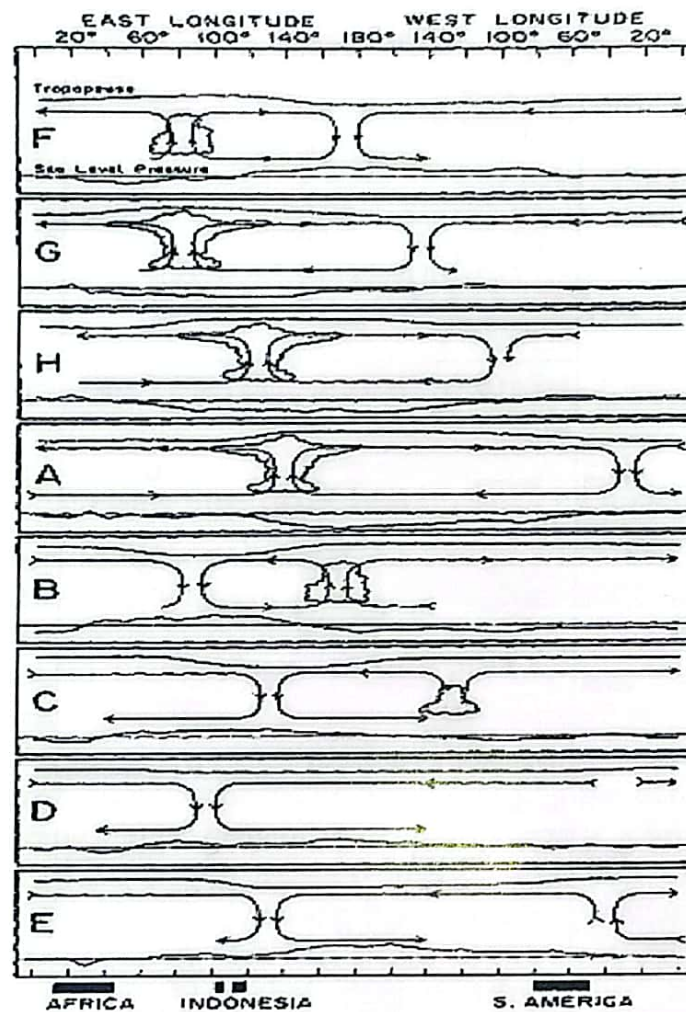
Gambar 2-1a: Skema sirkulasi MJO 40-50 harian yang dipengaruhi oleh angin zonal. Periode sirkulasi MJO disimbolkan dengan huruf di atas dimana skema konveksi kuat ditandai oleh terbentuknya awan cumulus dan cumulonimbus (Madden dan Julian, 1972)
