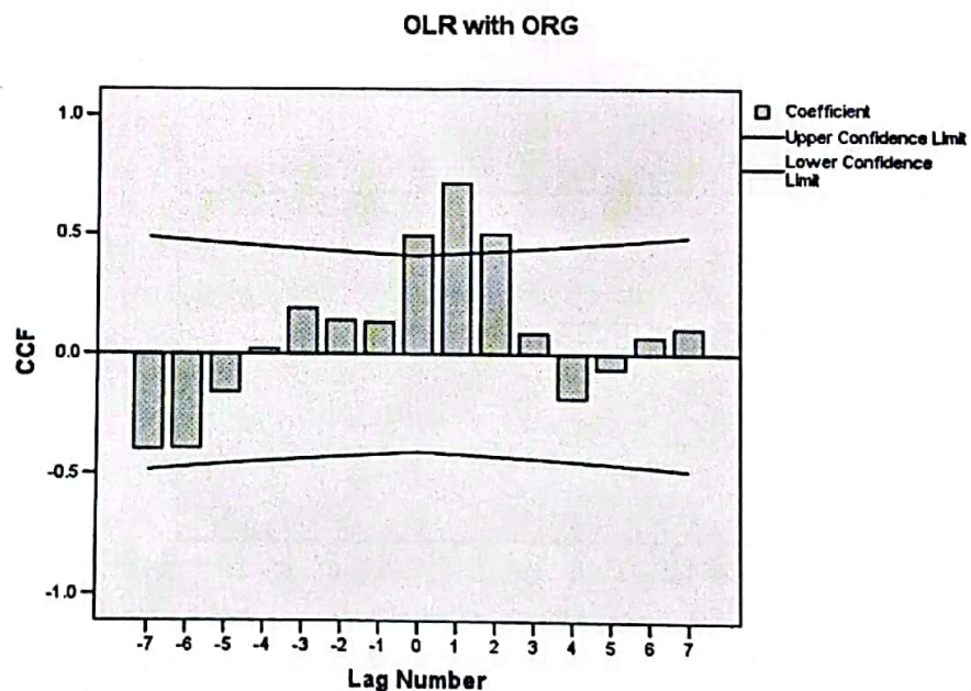
Gambar 4-3b: Grafik korelasi silang OLR-curah hujan (ORG) Kototabang pada 1 Maret - 30 Juni 2004
