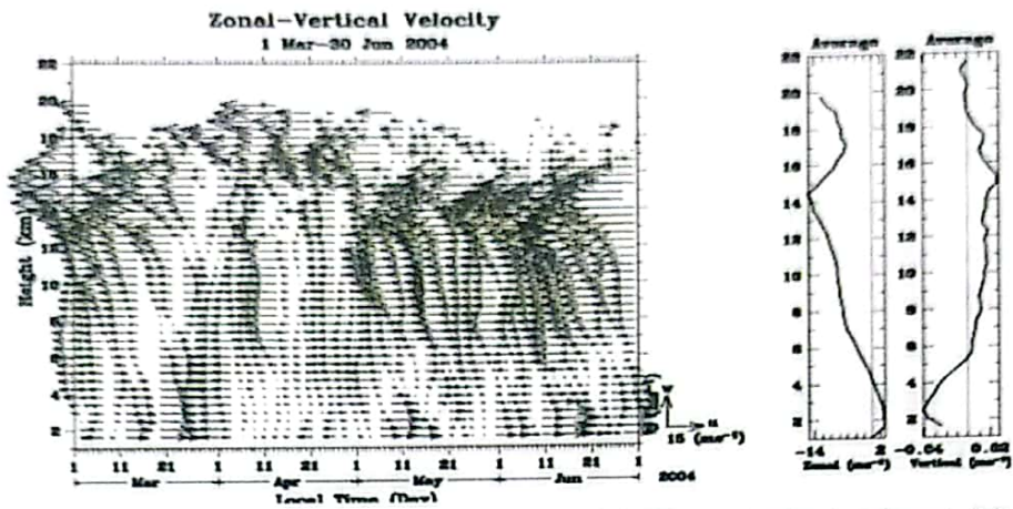
Gambar 4-1b: Vektor angin zonal-vertical EAR periode 1 Maret-30 Juni 2004
