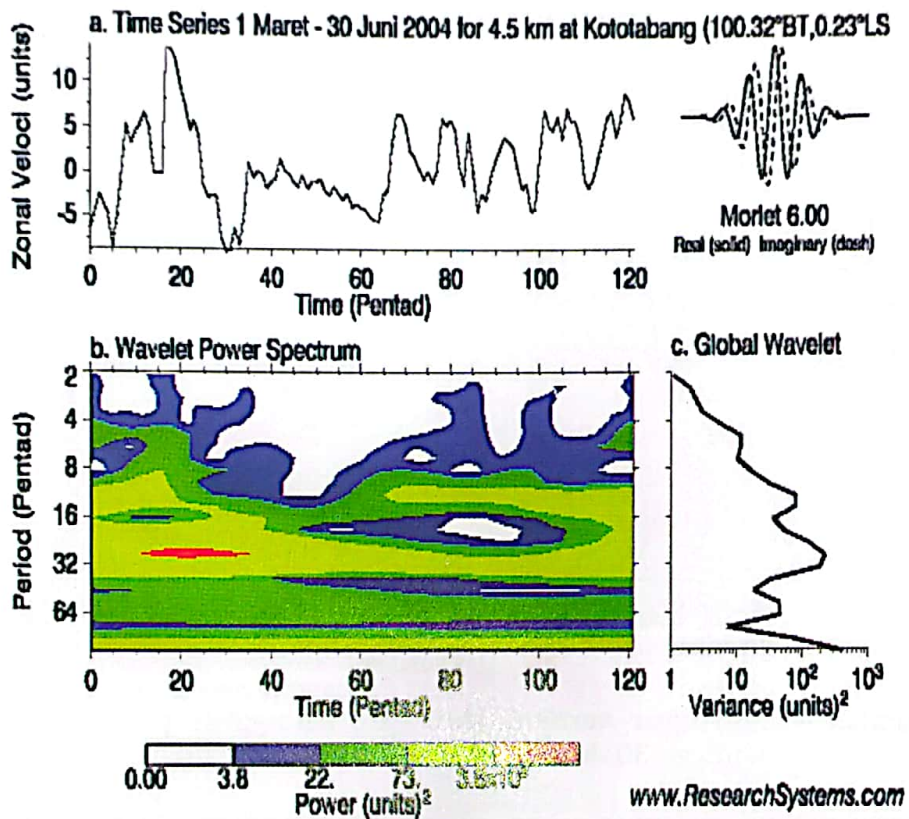
Gambar 4-1f: Sama dengan Gambar 4-1e, tetapi dengan teknik wavelet
