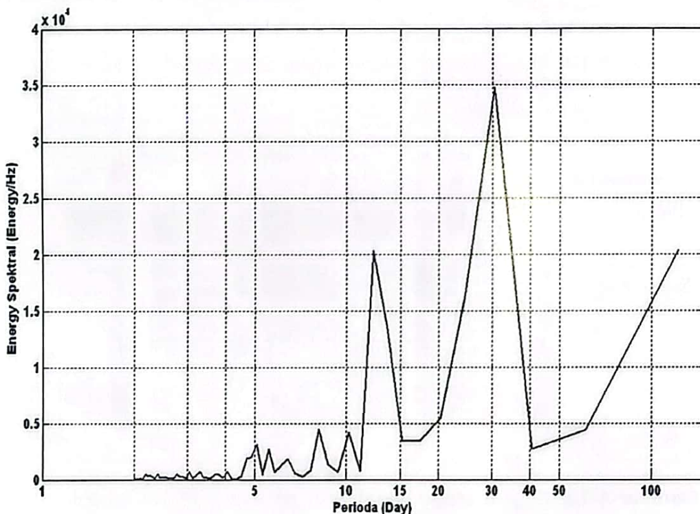
Gambar 4-1e: Energi Spektral angin zonal EAR periode 1 Maret-30 Juni pada ketinggian 4.5 km, dimana terlihat adanya osilasi kuat sekitar 30 harian
