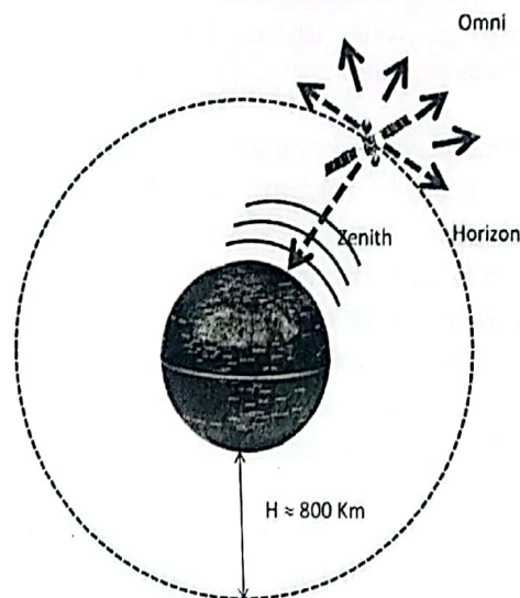
Gambar 3-1: Teknik perekaman data partikel oleh satelit NOAA 15
