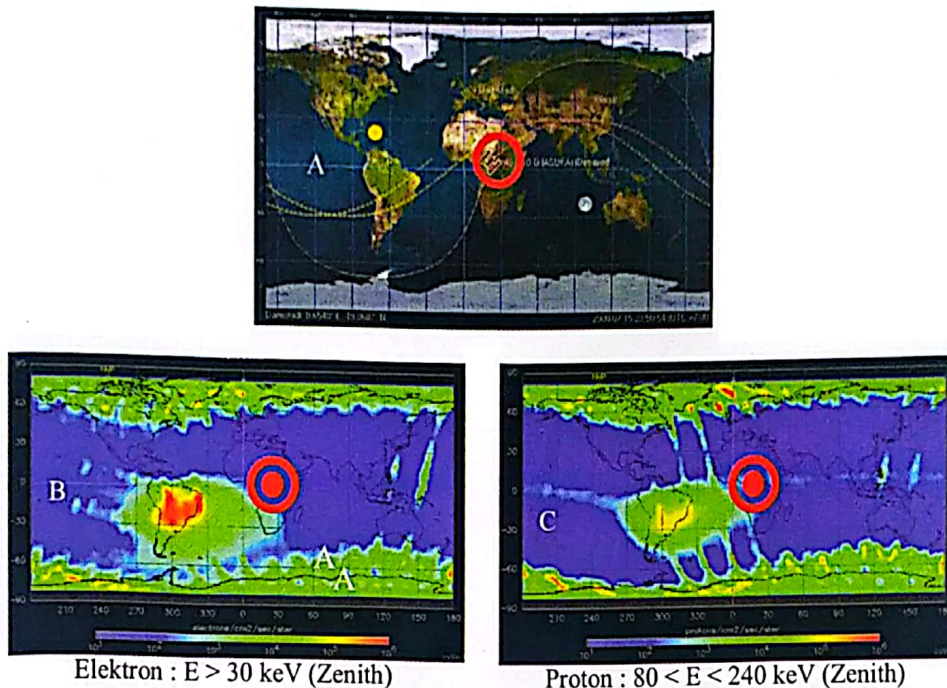
Gambar 4-2: Distribusi partikel saat anomali satelit ERS1
