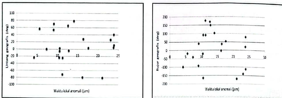
Gambar 4-5: Posisi lintang (kiri) dan bujur (kanan) geografis anomali satelit
