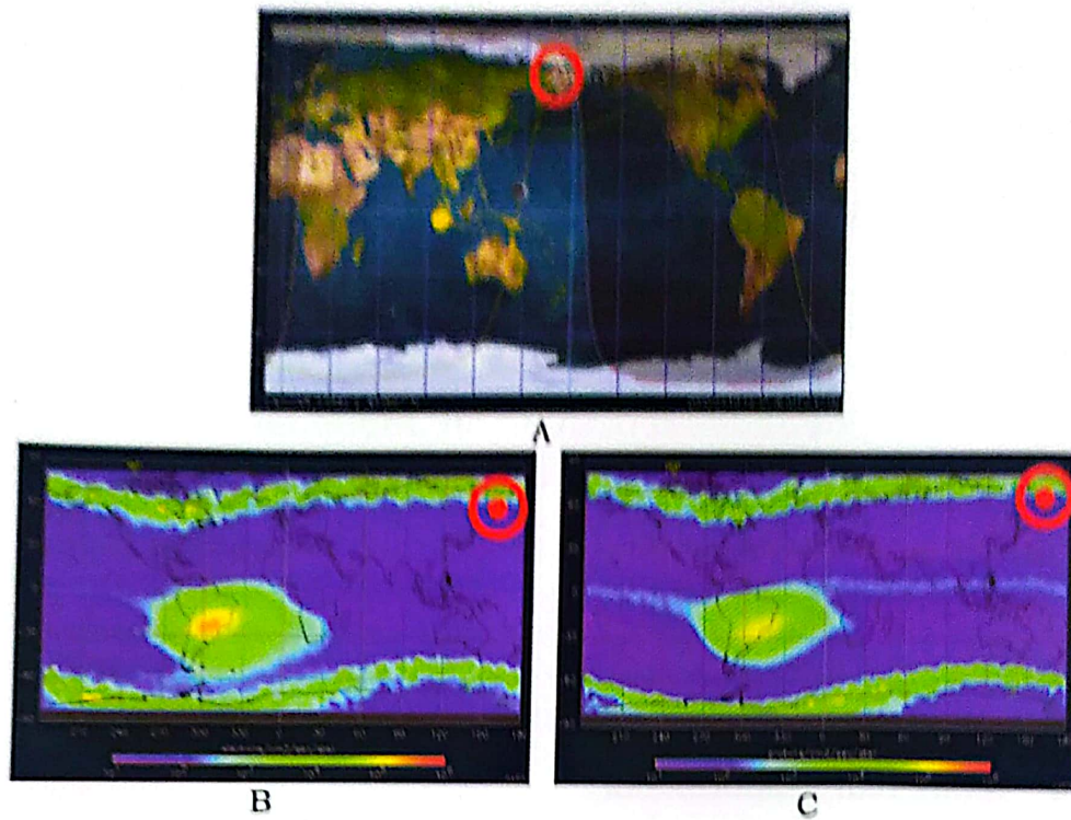
Gambar 4-1: Distribusi partikel saat anomali satelit ERS1
