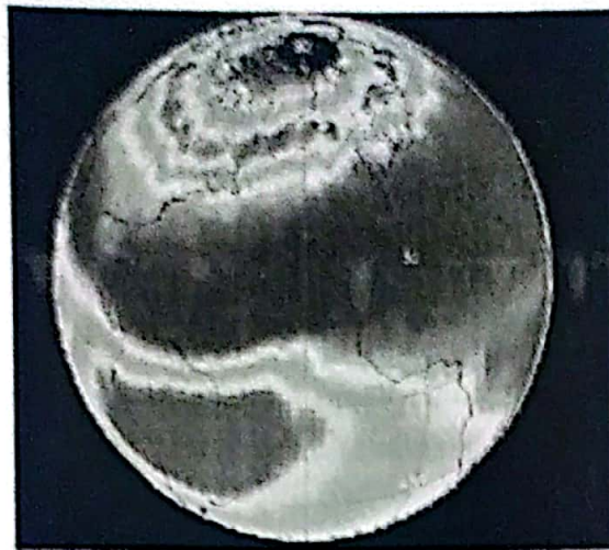
Gambar 4-8: Akumulasi partikel di daerah kutub
