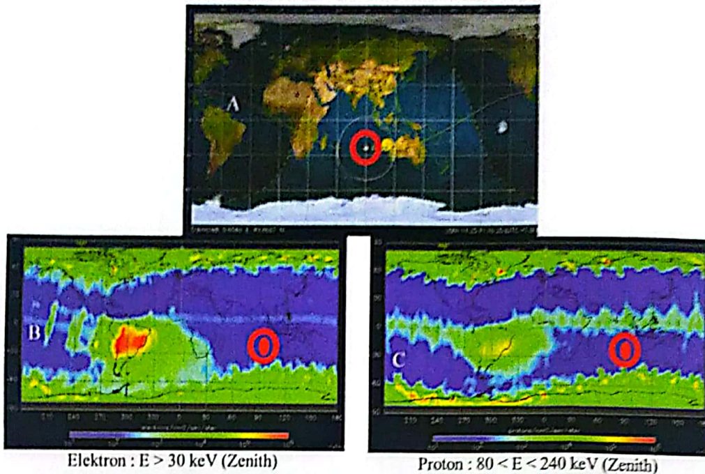
Gambar 4-3: Distribusi partikel saat anomali satelit FUSE (1)
