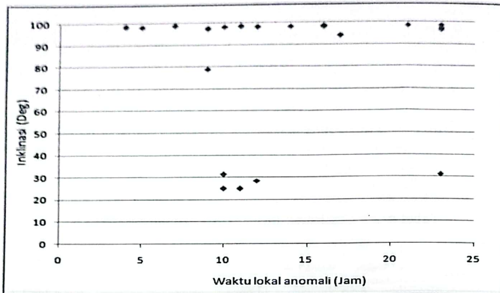
Gambar 4-7: Distribusi anomali satelit berdasarkan inklinasi
