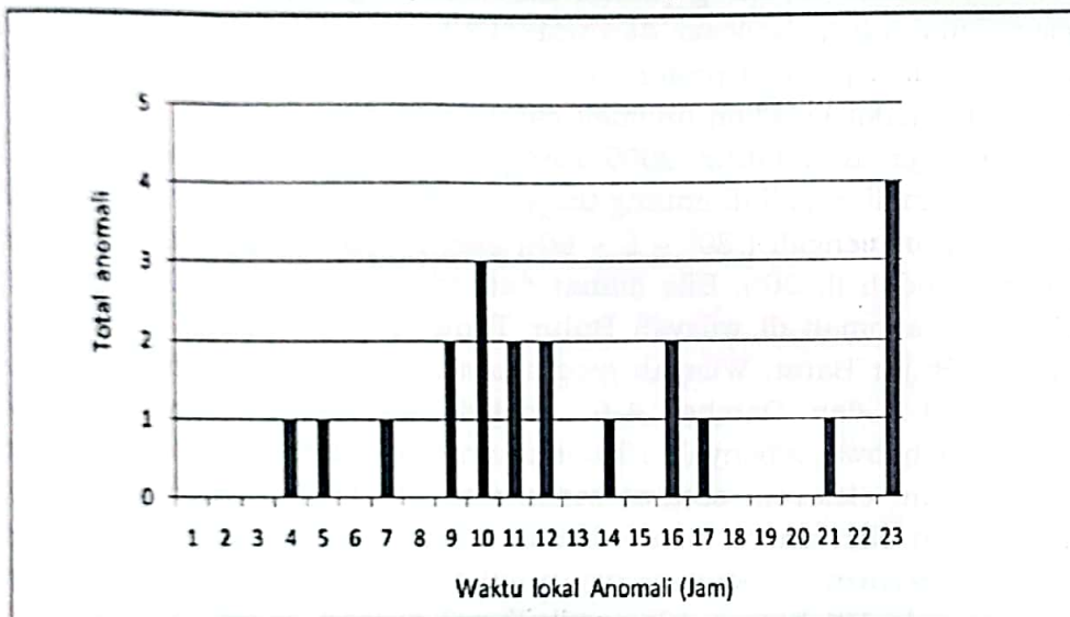
Gambar 4-9: Waktu lokal anomali satelit
