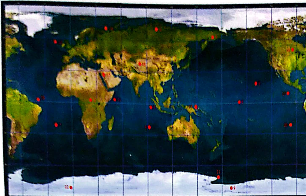
Gambar 4-6: Lokasi anomali satelit orbit rendah pada peta dunia
