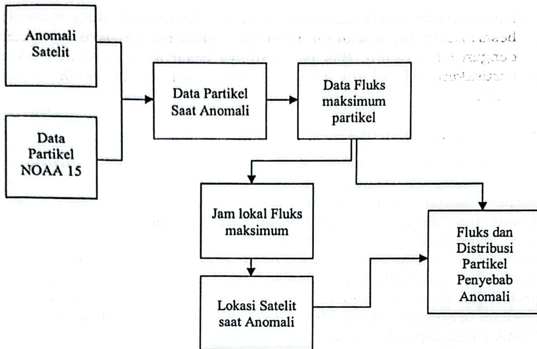
Gambar 2-1: Diagram metode untuk mengetahui tingkat fluks dan distribusi partikel penyebab anomali satelit
