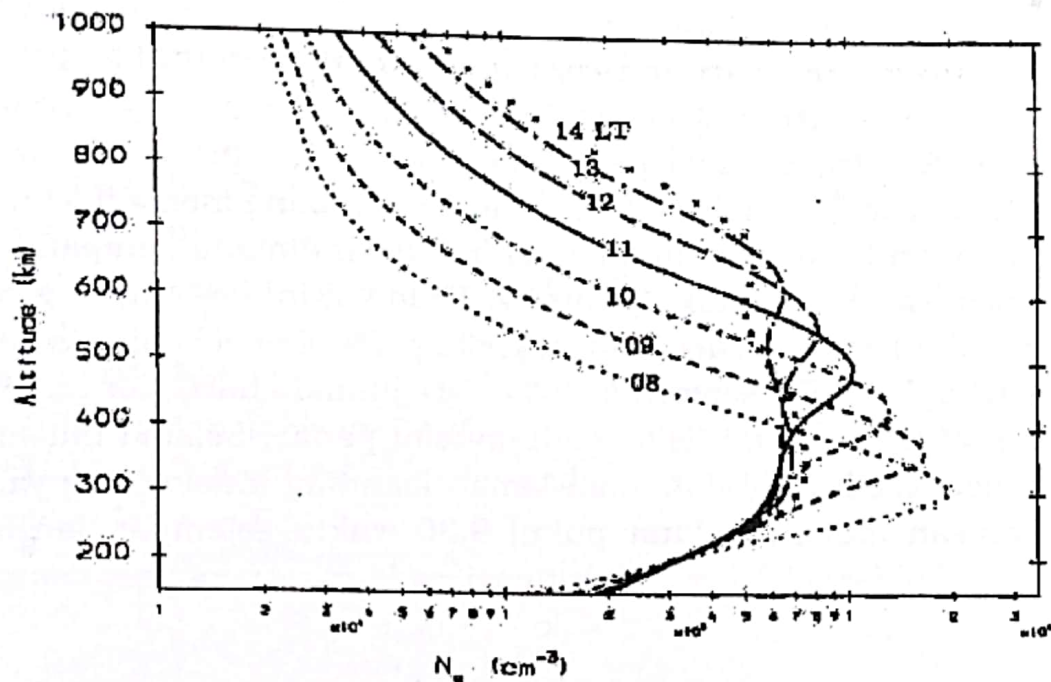
Gambar 2-1: Model profil kerapatan elektron untuk bujur Fortaleza dalam kondisi lapisan F3 paling kuat. (Balan dkk, 1998)
