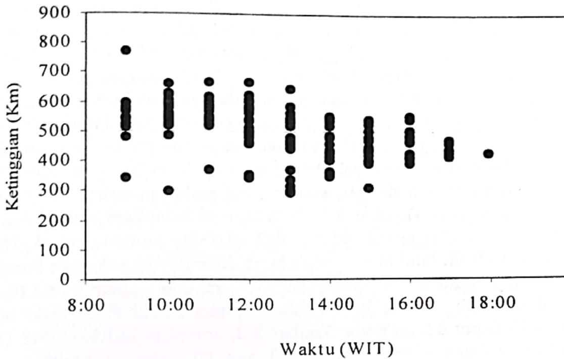
Gambar 3-4: Ketinggian lapisan F3
