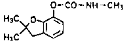
Struktur kimia Karbofuran ((2,3-dihidro-2,2-dimetil-7-benzofuranil metil karbamat)
