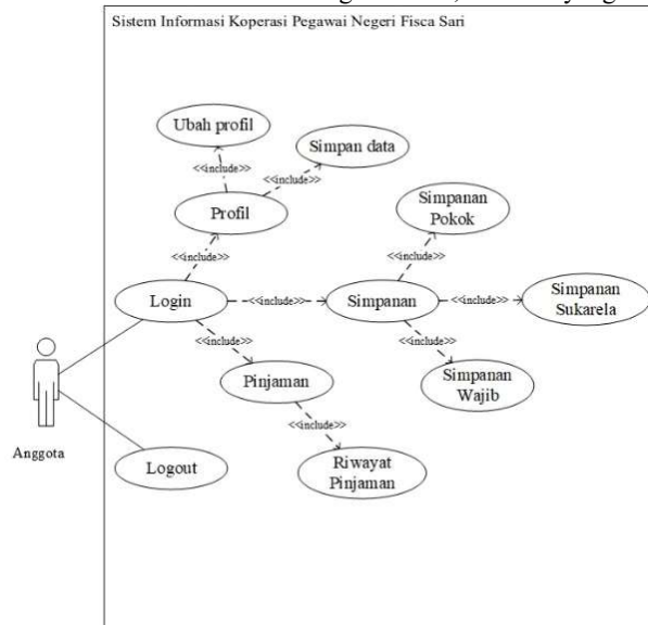
Gambar 3. Use case diagram anggota
