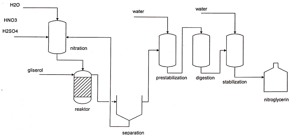
Gambar 1-1: Diagram alir proses pembuatan nitroglycerin
