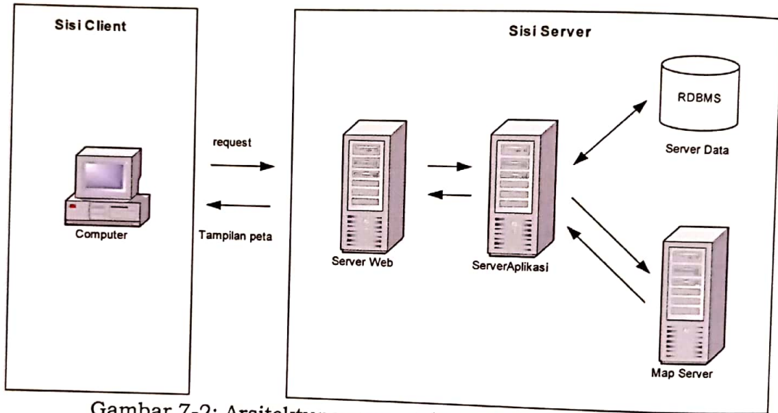
Gambar 7-2: Arsitektur umum aplikasi pemetaan di Web
