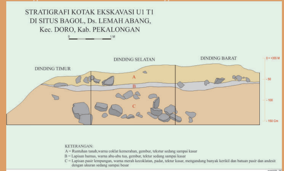
Gambar 3 : Stratigrafi lapisan tanah Candi Lemah Abang
