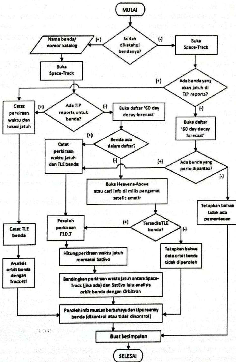
Gambar 5-1: Diagram alir prosedur pemantauan benda jatuh antariksa
