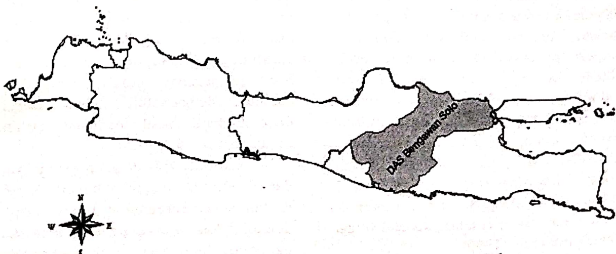
Gambar 2-1: Daerah kajian analisis DAS Bengawan Solo
