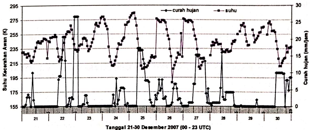
Gambar 3-1: Deret waktu suhu kecerahan awan dari MTSAT dan curah hujan dari QMorph periode tanggal 21-30 Desember 2007 jam 00-23 UTC di wilayah DAS Bengawan Solo
