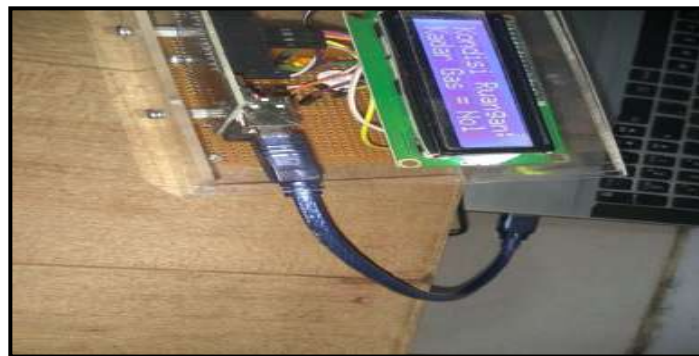
Gambar 7. Arduino Uno di hubungkan dengan Laptop
