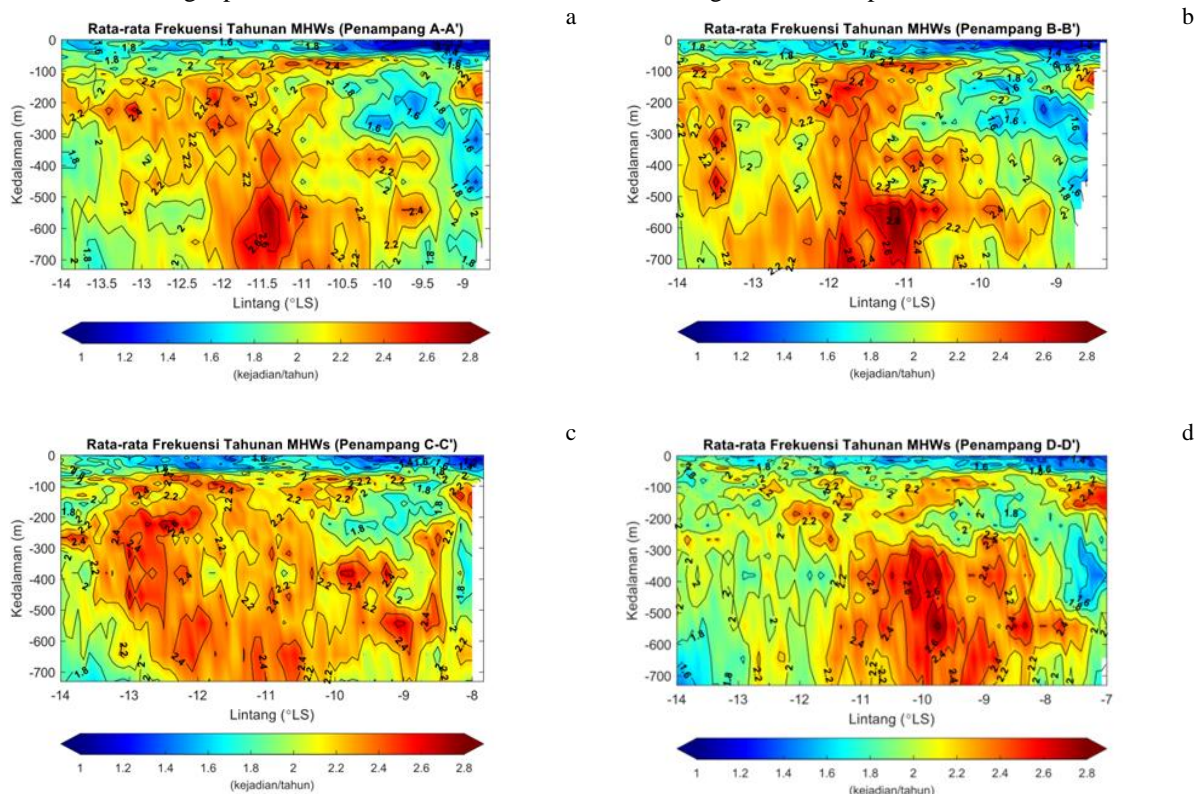
Gambar 3. Rata-rata Frekuensi Kejadian Tahunan MHWs selama 27 Tahun pada Kedalaman 0,4-763m. (a) Penampang AA', (b) Penampang BB', (c) Penampang CC', dan (d) Penampang DD'
