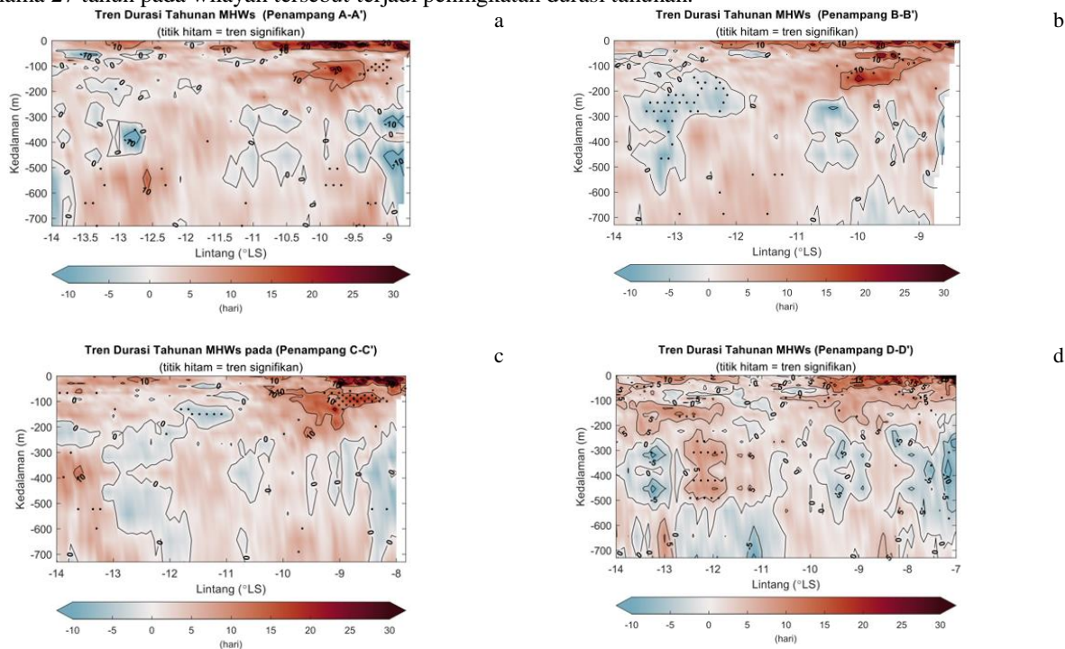
Gambar 7. Tren Durasi Tahunan Kejadian MHWs selama 27 Tahun pada Kedalaman 0,4-763m. (a) Penampang AA', (b) Penampang BB', (c) Penampang CC', dan (d) Penampang DD'
