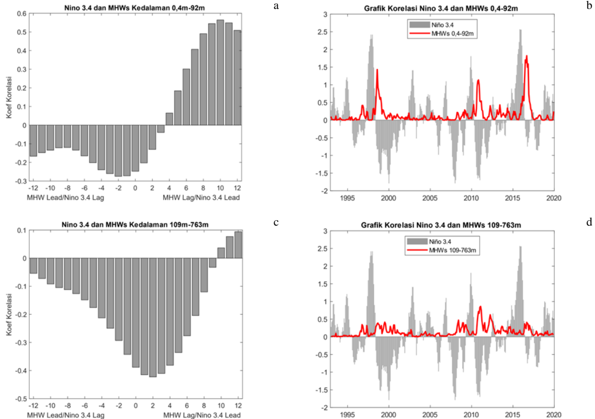
Gambar 9. Korelasi Antara Kejadian ENSO dengan Kejadian MHWs. (a) Korelasi silang pada kedalaman 0,4-92m, (b) Grafik korelasi pada kedalaman 0,4-92m, (c) Korelasi silang pada kedalaman 109-763m, dan (d) Grafik korelasi pada kedalaman 109-763m
