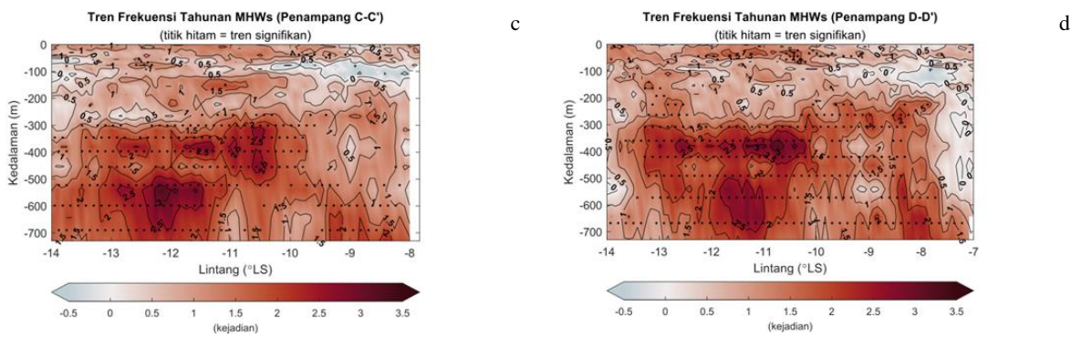
Gambar 6. Tren Frekuensi Kejadian Tahunan MHWs selama 27 Tahun pada Kedalaman 0,4-763m. (a) Penampang AA', (b) Penampang BB', (c) Penampang CC', dan (d) Penampang DD'
