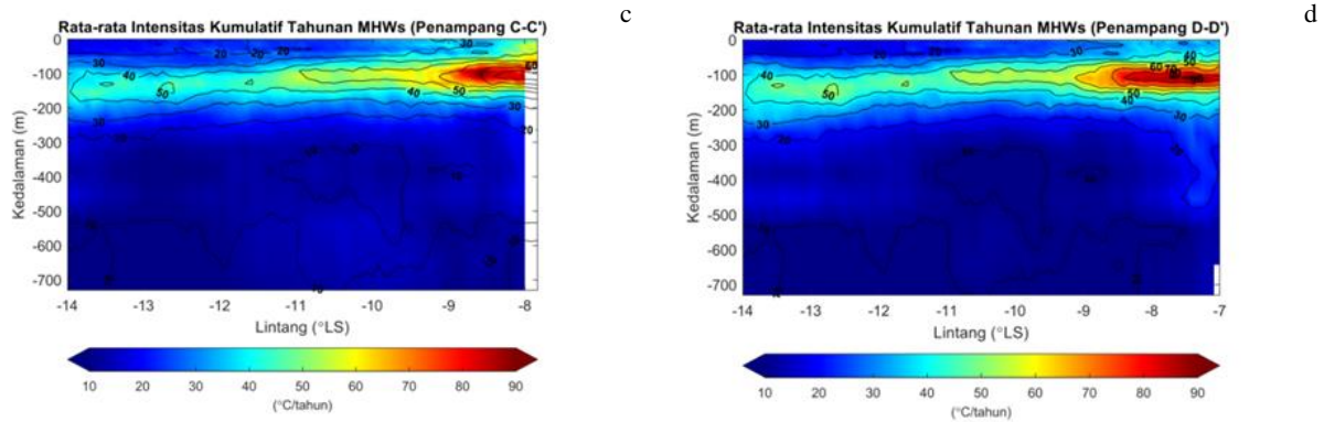
Gambar 5. Rata-rata Intensitas Kumulatif Kejadian Tahunan MHWs selama 27 Tahun pada Kedalaman 0,4-763m. (a) Penampang AA', (b) Penampang BB', (c) Penampang CC', dan (d) Penampang DD'
