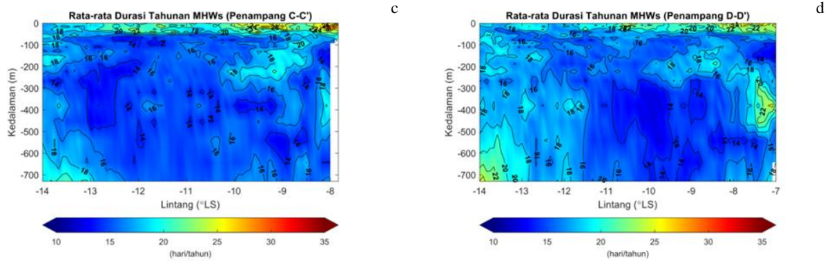
Gambar 4. Rata-rata Durasi Tahunan Kejadian MHWs selama 27 Tahun pada Kedalaman 0,4-763m. (a) Penampang AA', (b) Penampang BB', (c) Penampang CC', dan (d) Penampang DD'
