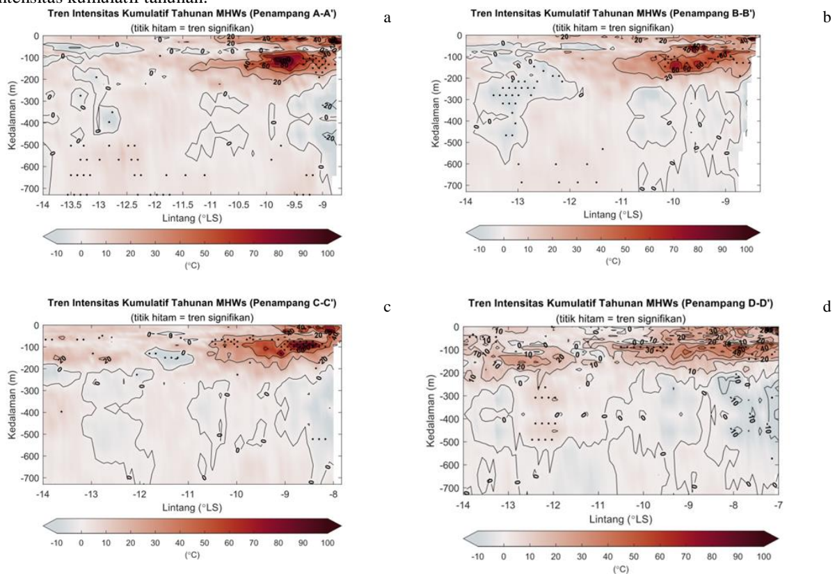
Gambar 8. Tren Intensitas Kumulatif Tahunan Kejadian MHWs selama 27 Tahun pada Kedalaman 0,4-763m. (a) Penampang AA', (b) Penampang BB', (c) Penampang CC', dan (d) Penampang DD'
