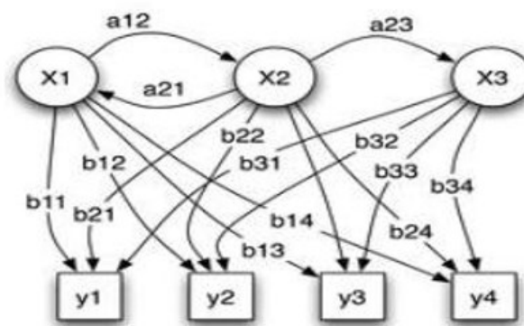
Gambar 2. Representasi dari parameter HMM yang digunakan [1]
