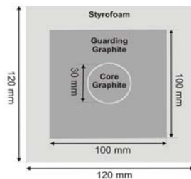
Gambar 2. Perangkat inti grafit tampak atas
