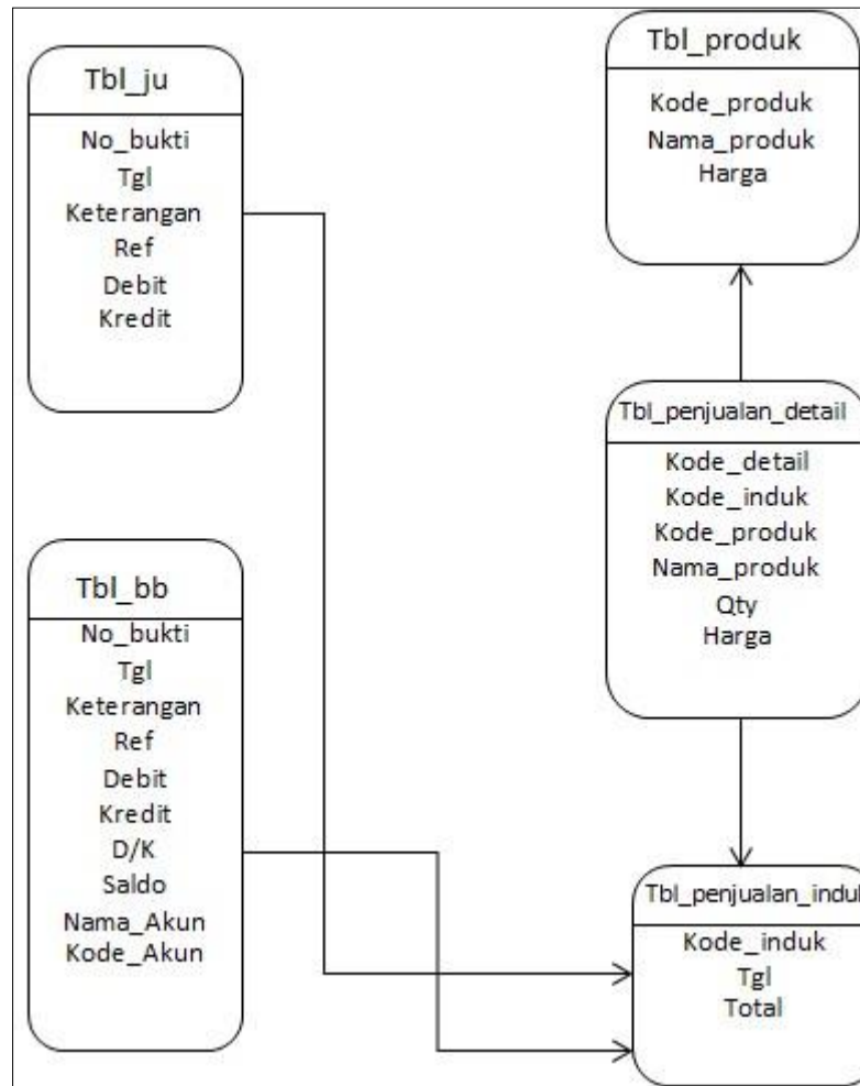
Gambar 2. ERD
