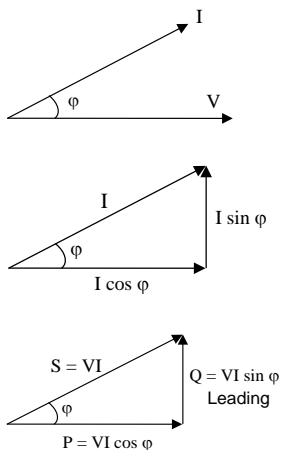
Gambar 15. Segitiga Daya untuk beban Kapasitif
