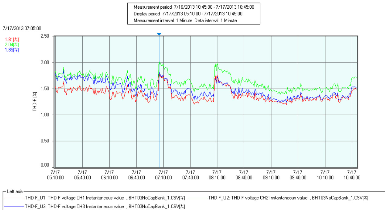
Gambar 11. THD tegangan masing-masing fasa
