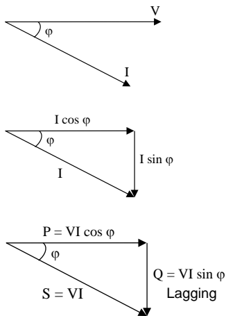
Gambar 14. Segitiga Daya untuk beban induktif
