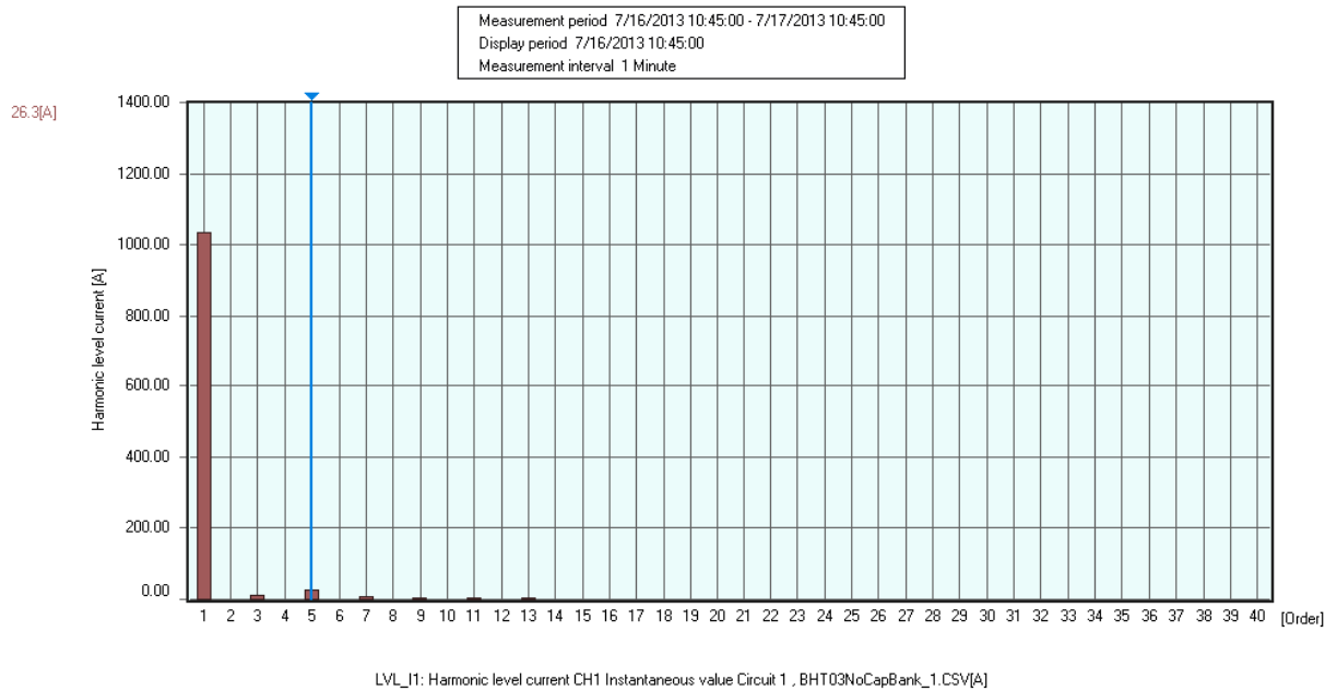
Gambar 6. Profil Harmonisa arus fasa R
