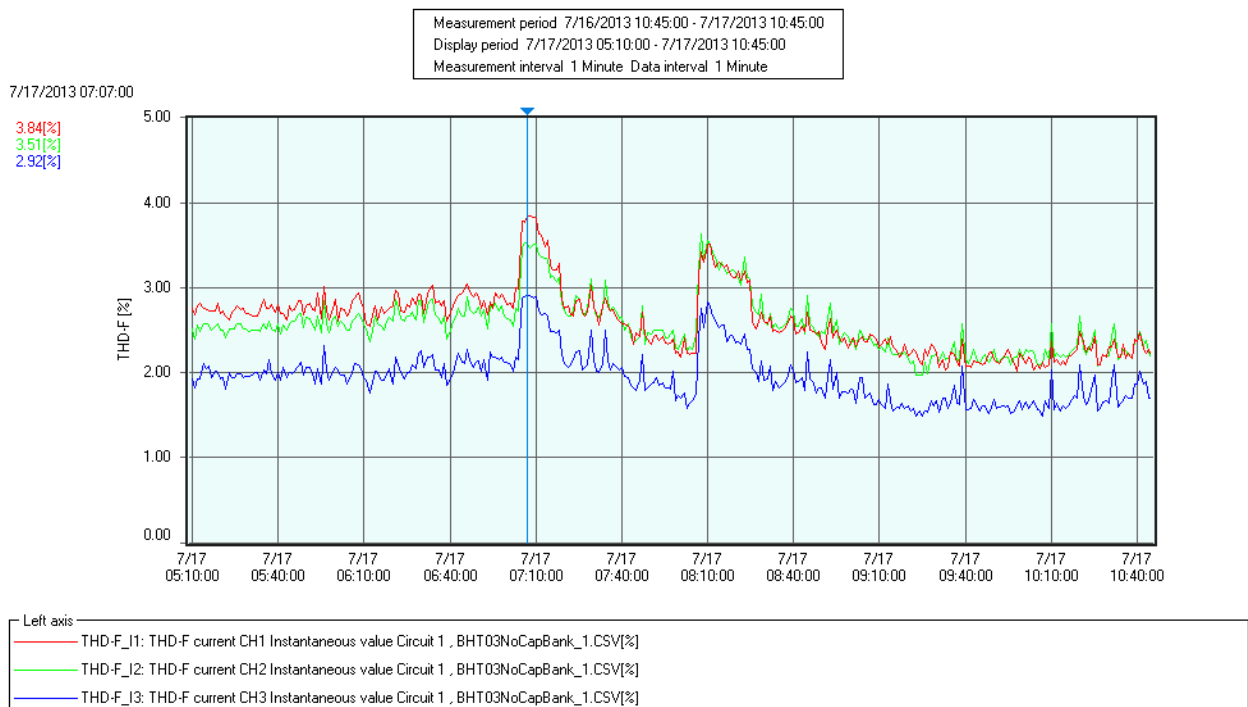
Gambar 11. THD arus masing-masing fasa
