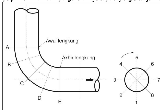
Gambar 6. Titik pengukuran konstruksi pipa elbow sebelum dan sesudah pompa
