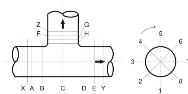
Gambar 5. Titik pengukuran konstruksi pipa T-Join
