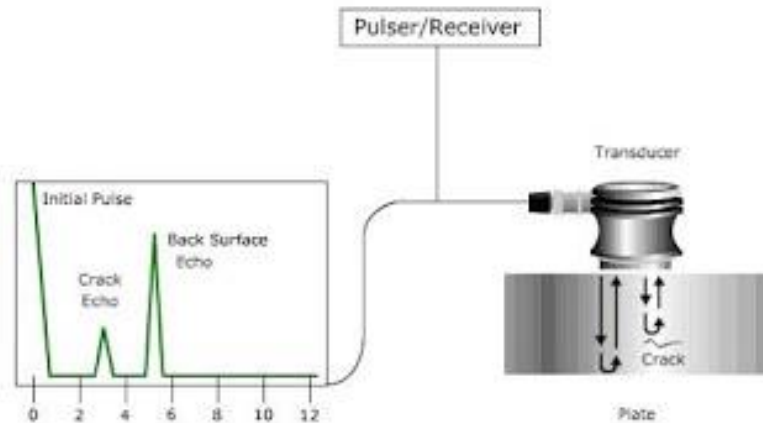
Gambar 1. Prinsip dasar uji ultrasonik
