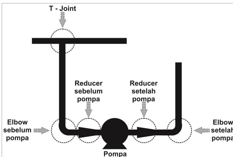
Gambar 9. Segmen/bagian pengukuran pipa pendingin primer RSG-GAS
