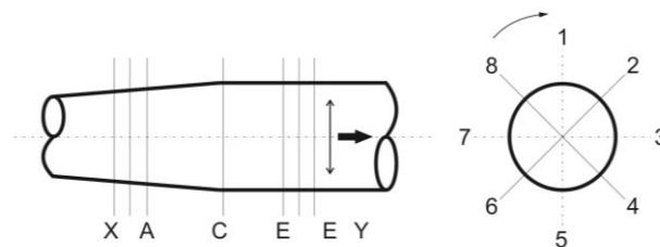
Gambar 7. Titik pengukuran konstruksi pipa reducer sebelum dan sesudah pompa
