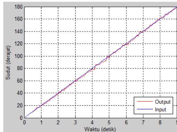
Gambar 3-2. Grafik pengujian input dan output tilt gimbal
