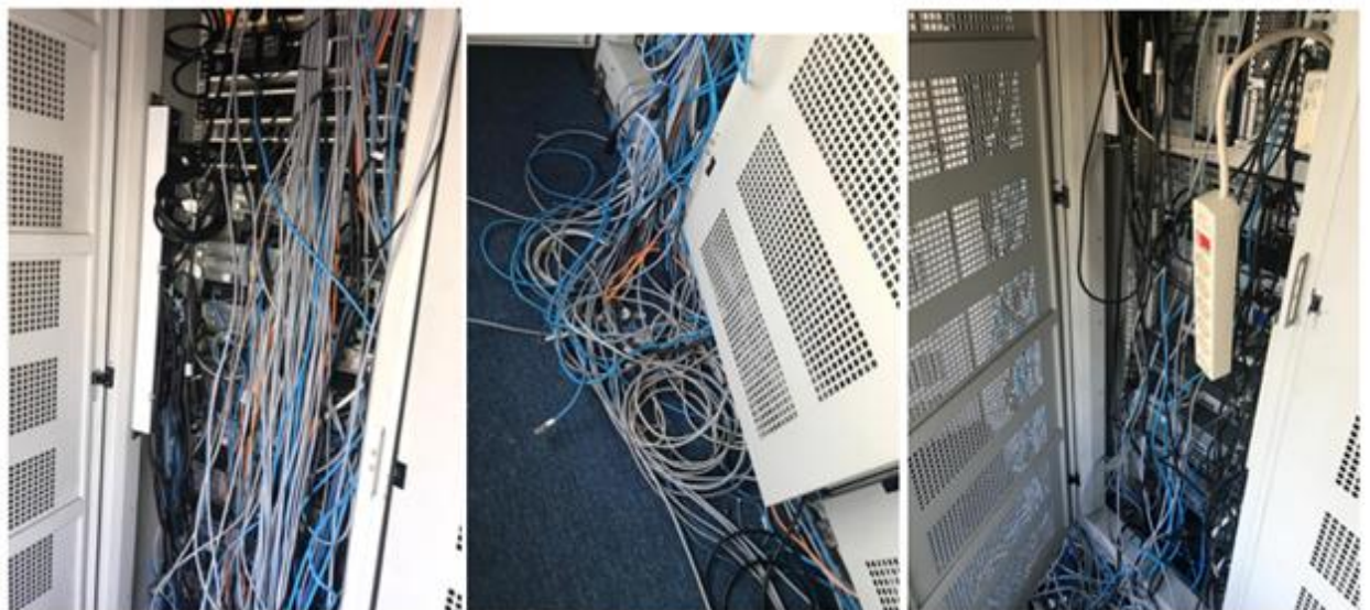
Gambar 2. Kondisi Kabel Sebelum dilakukan Perapihan
