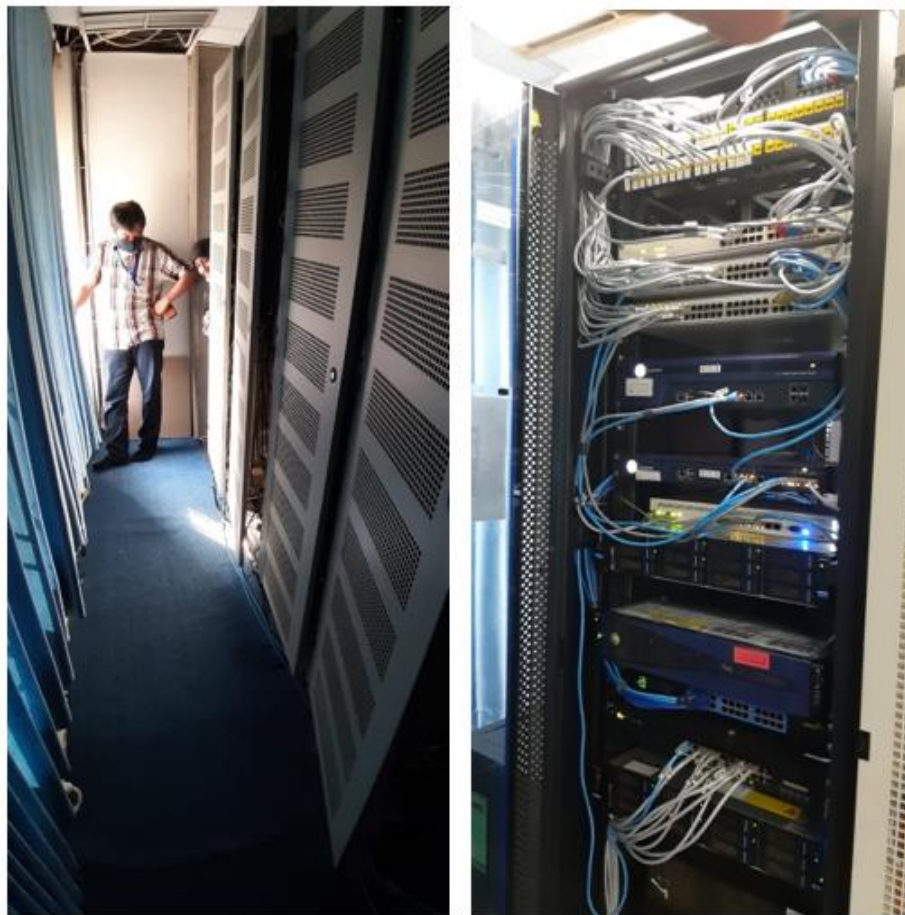
Gambar 4. Kondisi Kabel Setelah dilakukan Perapihan
