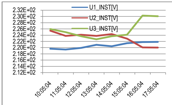
Gambar 5. Tegangan beban
