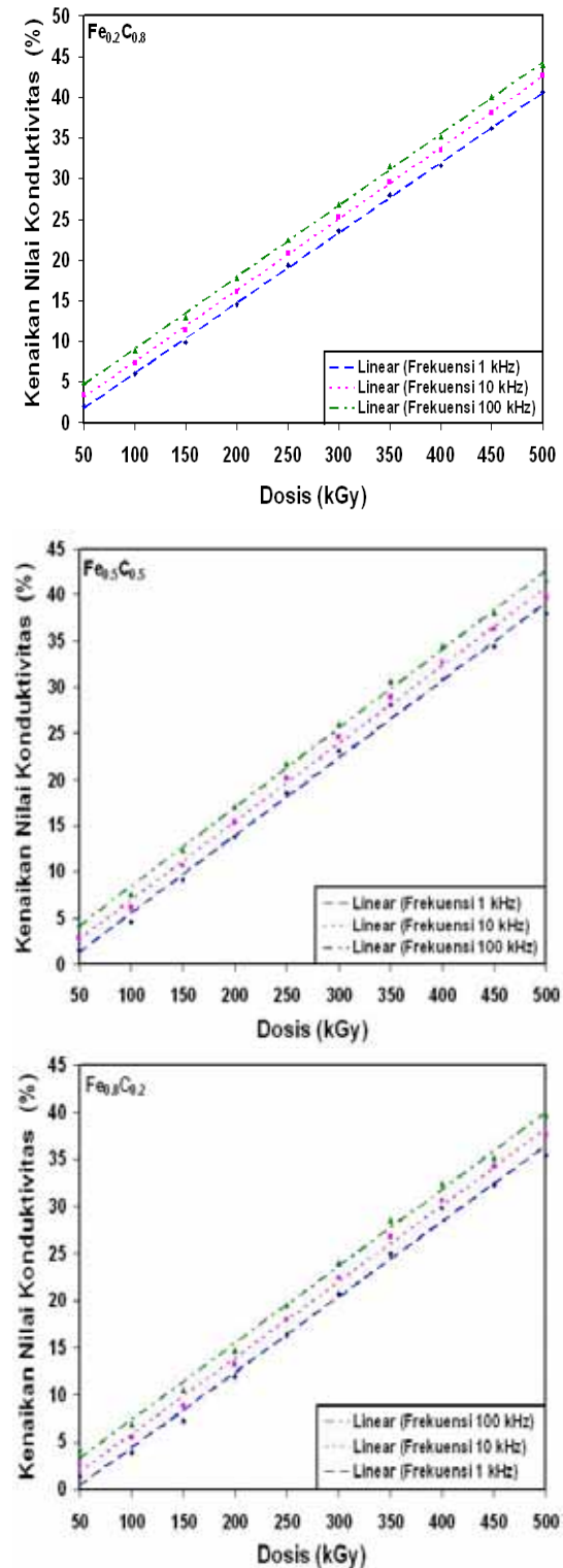
Gambar 1. Persentase peningkatan nilai konduktivitas bahan komposit Fe_xC_{1-x} oleh radiasi sinar- \gamma
