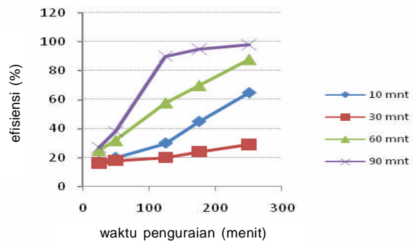
Gambar 6. Pengaruh waktu homogenisasi dan waktu penguraian terhadap efisiensi degradasi MB dengan metode fenton untuk Fe_3O_4 ( Aldrich ).
