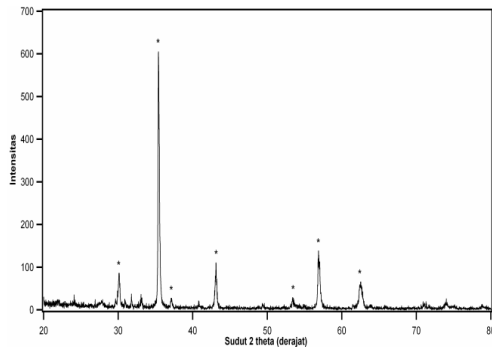
Gambar 2. Difraktogram pasir besi setelah dicuci dan dimilling
