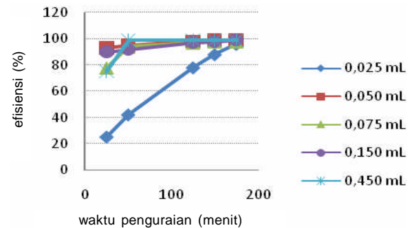
Gambar 13. Pengaruh konsentrasi H_2O_2 dan waktu penguraian terhadap efisiensi degradasi MB dengan metode fenton untuk katalis HSM.
