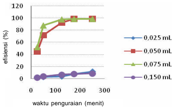
Gambar 7. Pengaruh konsentrasi H 2 O 2 dan waktu penguraian terhadap efisiensi degradasi MB dengan metode fenton untuk Fe 3 O 4 (Aldrich).
