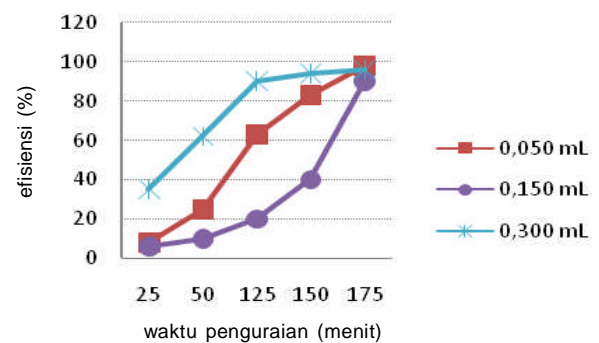
Gambar 14. Pengaruh konsentrasi H_2O_2 dan waktu penguraian terhadap efisiensi degradasi MB dengan metode fenton untuk katalis pasir besi.
