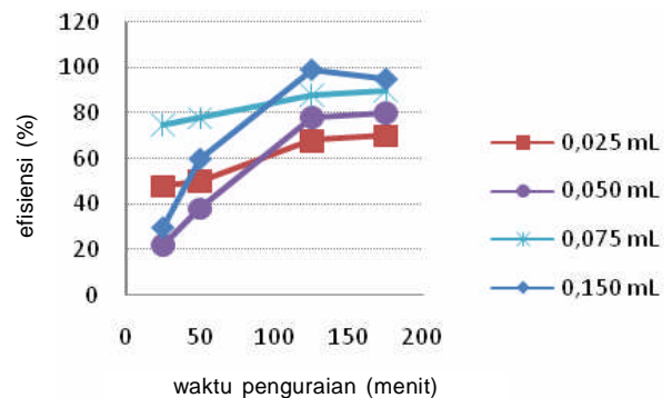
Gambar 8. Pengaruh konsentrasi H 2 O 2 dan waktu penguraian terhadap efisiensi degradasi MB dengan metode foto fenton untuk Fe 3 O 4 (Aldrich).
