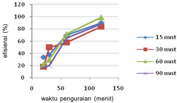
Gambar 9. Pengaruh waktu homogenisasi dan waktu penguraian terhadap efisiensi degradasi MB dengan metode foto fenton untuk Fe_3O_4 (Aldrich).
