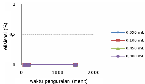
Gambar 5. Pengaruh konsentrasi H_2O_2 dan waktu penguraian terhadap efisiensi degradasi MB dengan metode fenton tanpa katalis Fe.
