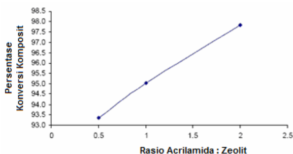
Gambar 9. Hubungan Antara Perbandingan Acrilamida Terhadap Zeolit dengan Persentase Konversi Komposit
