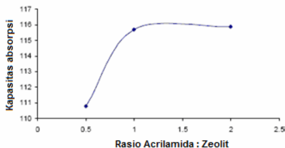
Gambar 10 Hubungan Antara Perbandingan Acrilamida Terhadap Zeolit dengan Kapasitas Absorpsi
