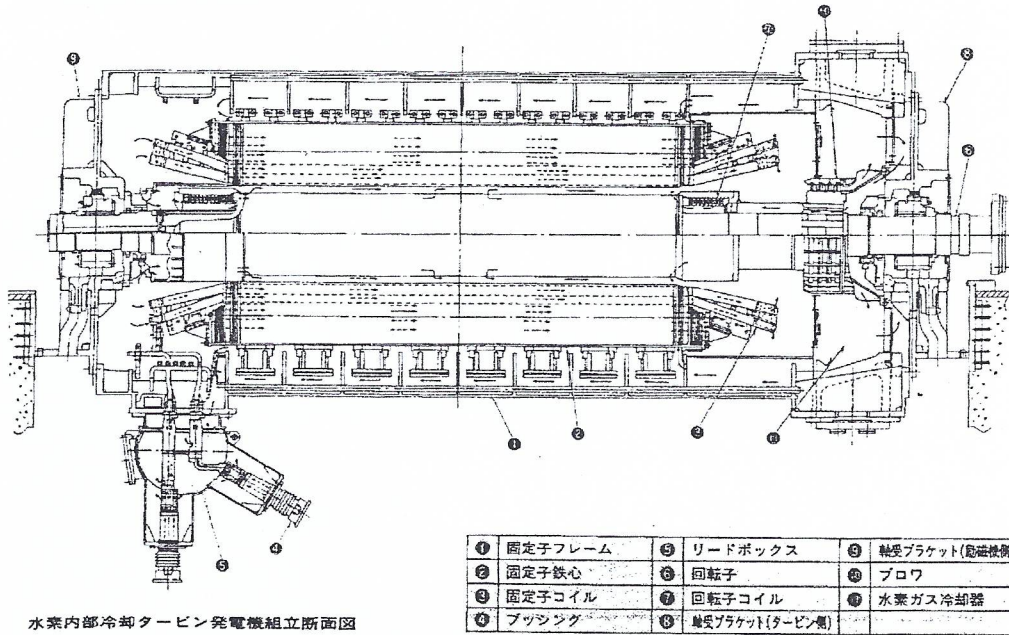
水素内部冷却タービン発電機組立断面図
