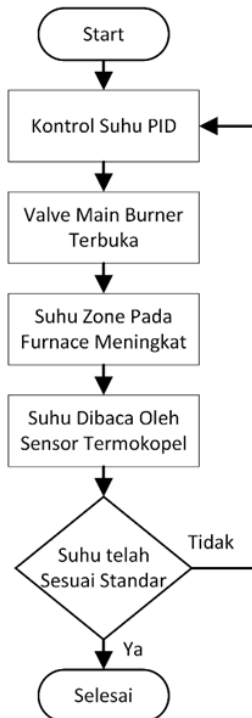
Gambar 5. Alur proses pengambilan data oleh sensor
