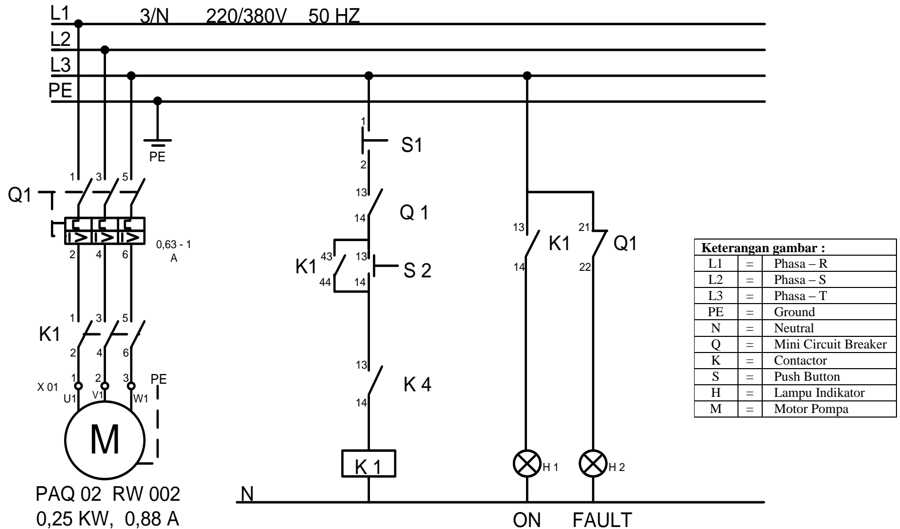
Gambar 4. Sistem kelistrikan mixer/pengaduk PAQ 02 RW 002
