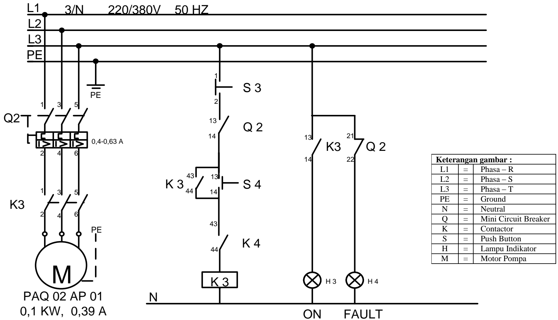
Gambar 2. Sistem kelistrikan pompa PAQ 02 AP01
