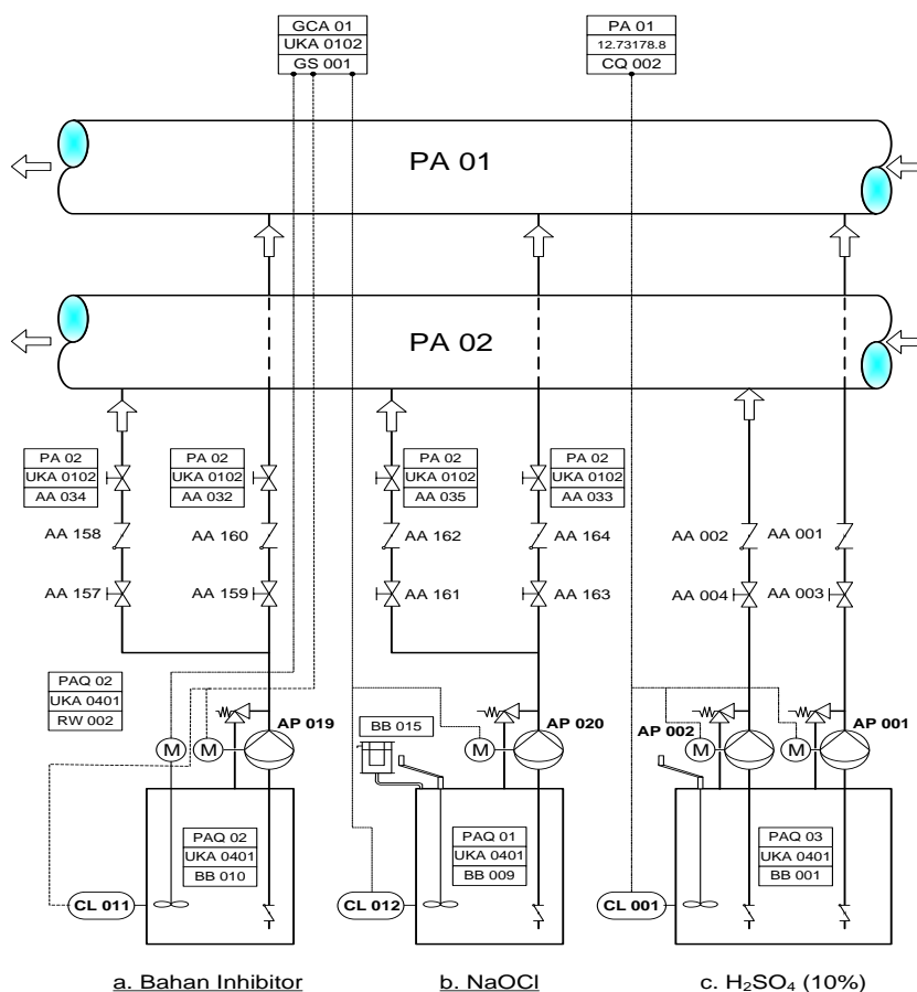
Gambar 1. Sistem Injeksi Bahan Kimia PAQ 01/02/03
