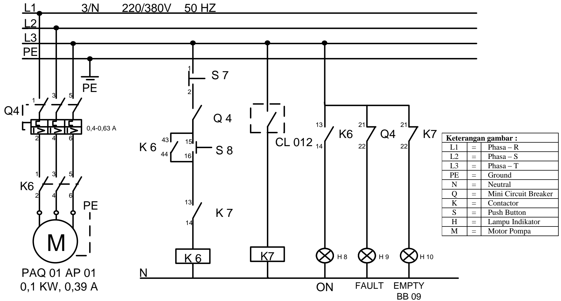
Gambar 5. Sistem kelistrikan Pompa PAQ 01AP 01
