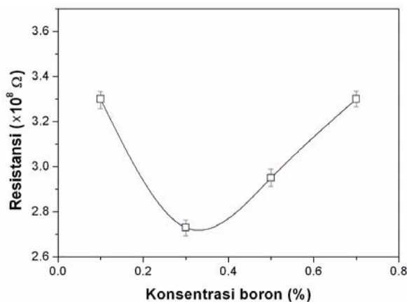
Gambar 2. Grafik resistansi vs konsentrasi Boron, pada tekanan gas 1,4 \times 10^{-1} Torr, suhu substrat 200^\circ\text{C} dan waktu deposisi 1,5 jam.
