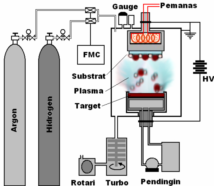
Gambar 1. Skema Peralatan Plasma Sputtering DC.
