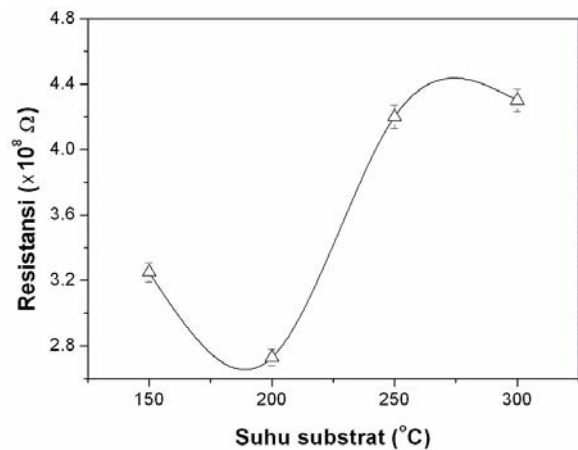
Gambar 3. Grafik resistansi vs suhu substrat, pada tekanan gas 1,4 \times 10^{-1} Torr, konsentrasi Boron 0,3 %, waktu deposisi 1,5 jam.
