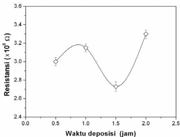
Gambar 4. Grafik resistansi vs waktu deposisi, pada tekanan gas 1,4 \times 10^{-1} Torr, suhu substrat 200 °C dan konsentrasi Boron 0,3 %.
