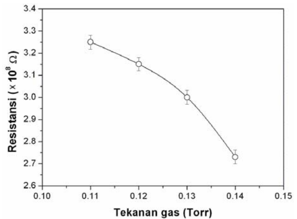
Gambar 5. Grafik resistansi vs tekanan gas, untuk waktu deposisi 1,5 jam, suhu substrat 200 °C, dan konsentrasi Boron 0,3 %.
